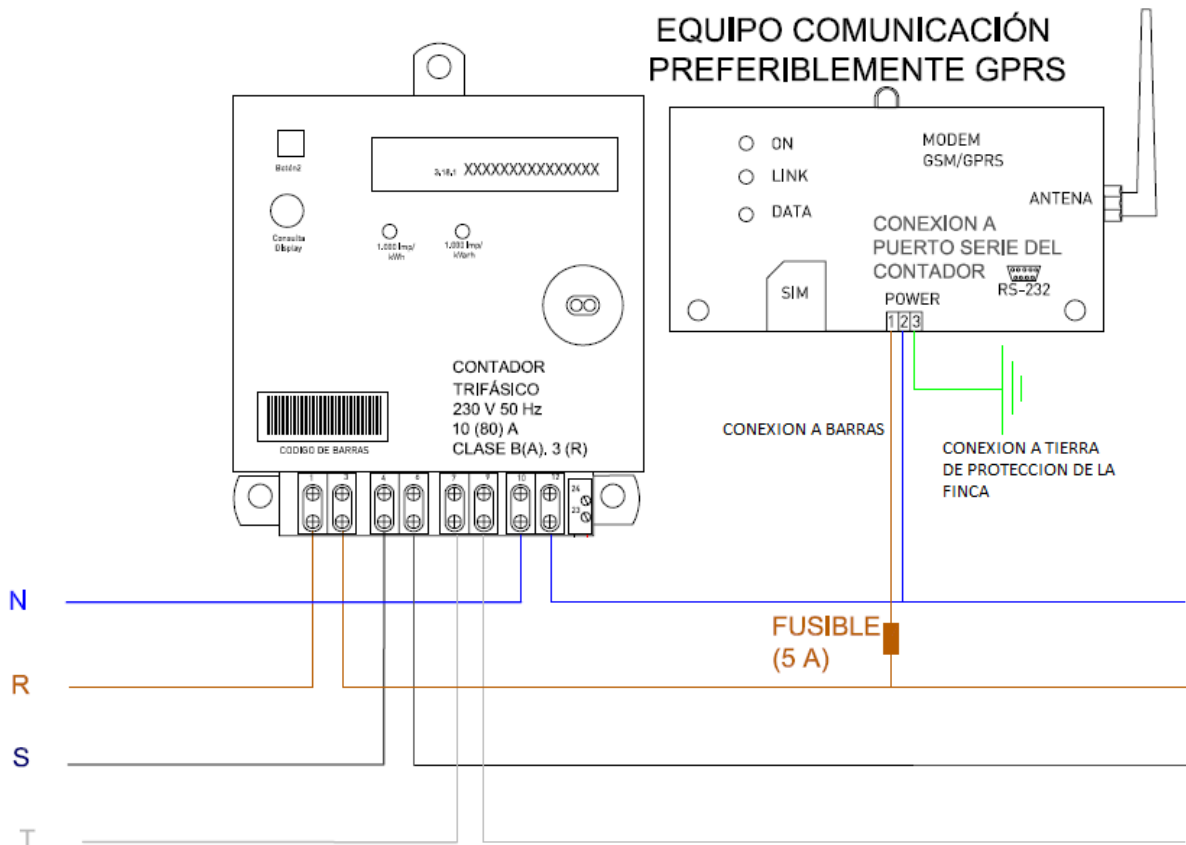
Figura 3. Instalación de medida directa en baja tensión (BT-DIR).
