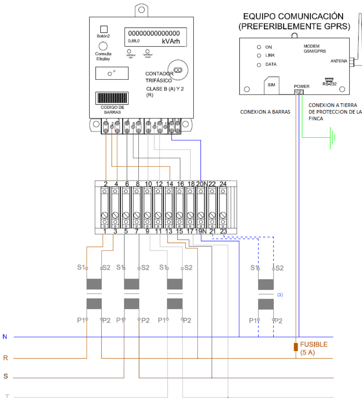
Figura 2. Instalación de medida indirecta en baja tensión (BT-IND).
