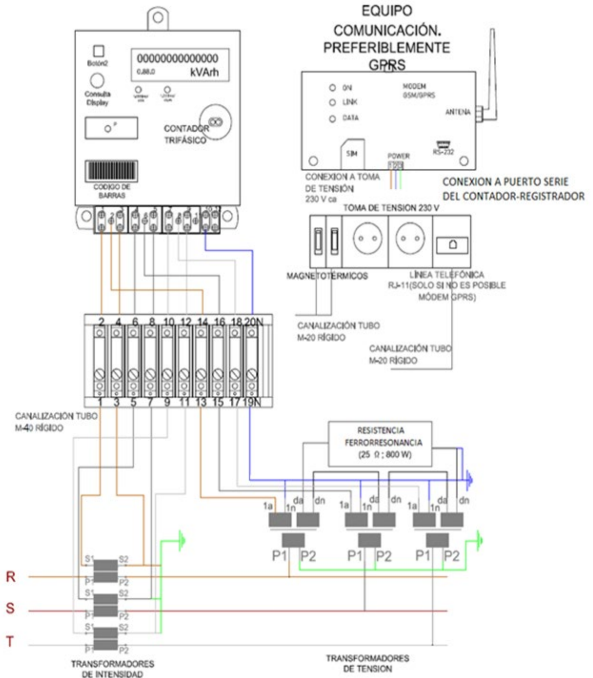
Figura 1. Instalación de medida en alta tensión de Un \leq 36\text{ kV} (MT-P).
