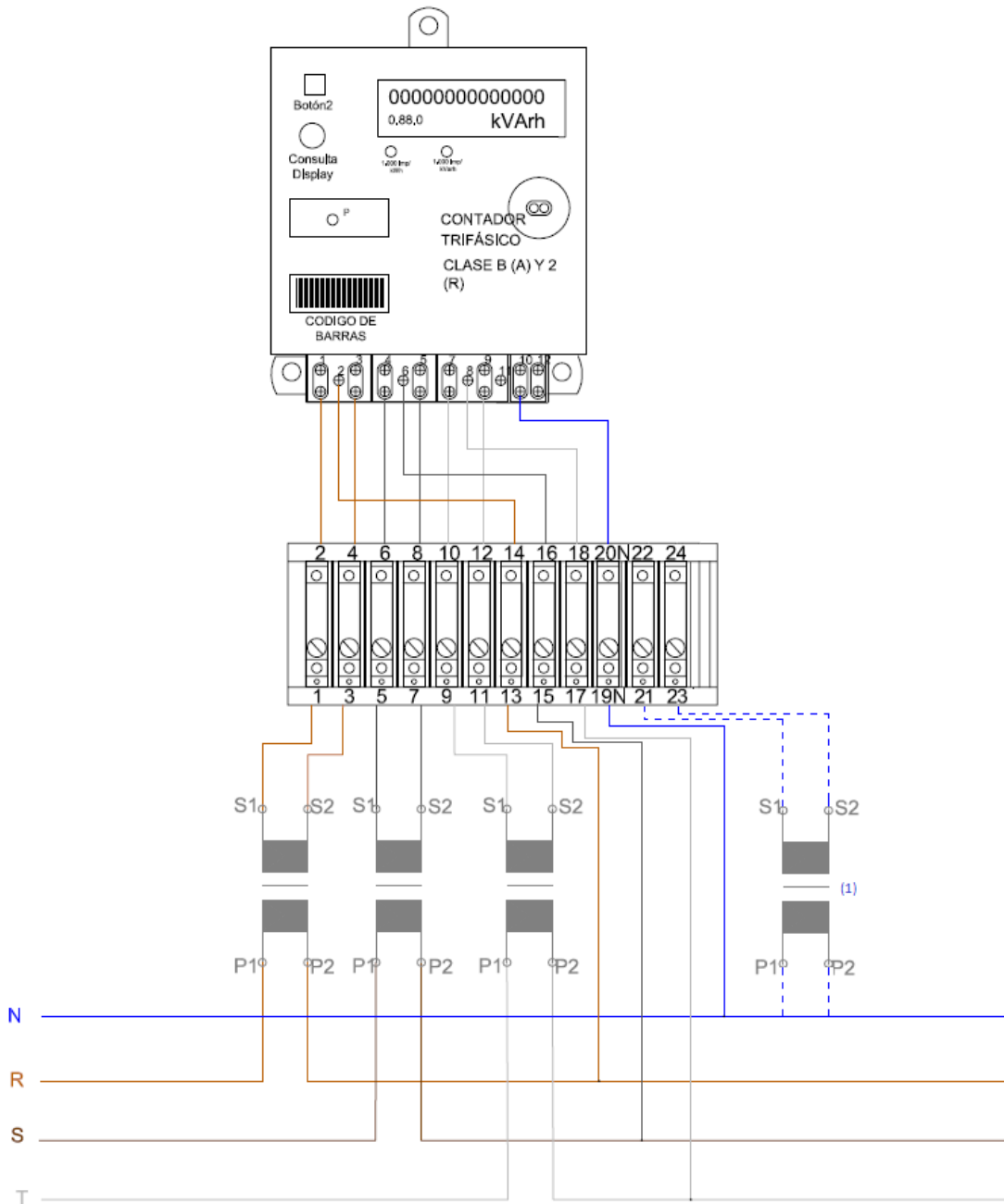
Figura 1. Instalación de medida Indirecta en baja tensión (BT-IND).
