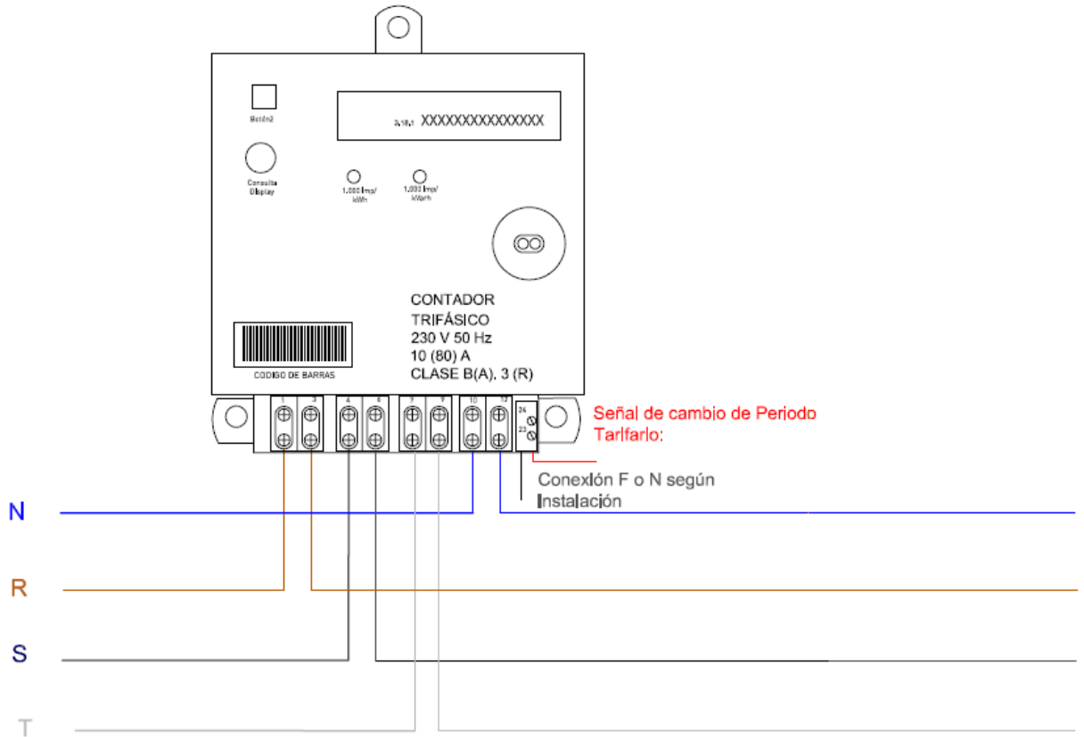
Figura 2. Instalación de medida directa trifásica en baja tensión (BT-DIR-III).
