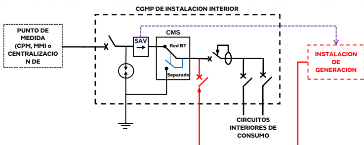
UBICACION DEL CMDS EN CGMP DE AUTOCONSUMOS INDIVIDUALES EN INSTALACION INTERIOR SIN EXCEDENTES
