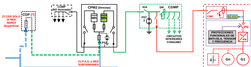
ESQUEMA 17 Individual - CON Compensación Excedentes - en CGMP Red interior - Generación (Renovable y mismo titular) - Finca 2 Suministros - P_{gII} \leq 50 \text{ kW} - P_{CG} \leq 50 \text{ kW} - Modo Dependiente
