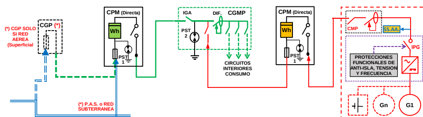
ESQUEMA 20 Individual - CON Venta Excedentes - en CGMP Red interior - Generación (NO Ren-Co-Res o Distinto Titular o Hibridación) - Finca 1 Suministro - P_{gII} \leq 50 \text{ kW} - P_{CG} \leq 50 \text{ kW} - Modo Dependiente
