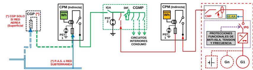
ESQUEMA 22 Individual - CON Venta Excedentes - en CGMP Red interior - Generación (NO Ren-Co-Res o Distinto Titular o Hibridación) - Finca 1 Suministro - 50 < P_{gII} \leq 100 \text{ kW} - PCG \leq 400 \text{ kW} - Modo Dependiente
