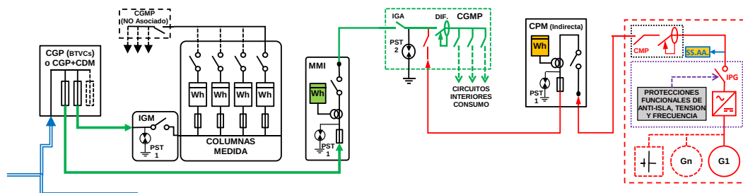
ESQUEMA 26 Individual - CON Venta Excedentes - en CGMP Red interior - Generación (NO Ren-Co-Res o Distinto Titular o Hibridación) - Finca \geq 2 Suministros - 50 < P_{gII} \leq 100 kW - PCG \leq 250 kW - Modo Dependiente
