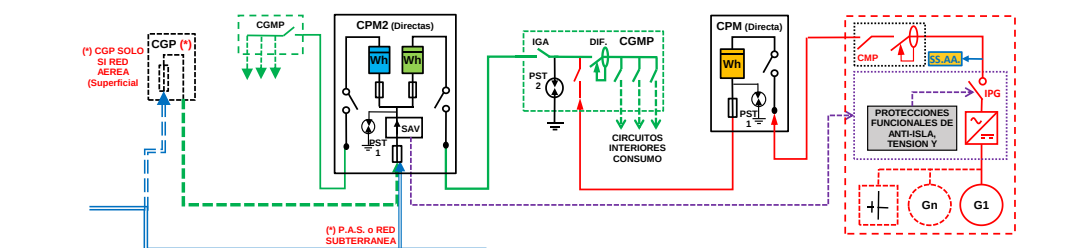
ESQUEMA 79 Colectivo - SIN Excedentes - en CGMP Red interior - Finca \geq 2 Suministros - P_{gII} \leq 50 kW - PCG \leq 50 kW - Modo Dependiente
