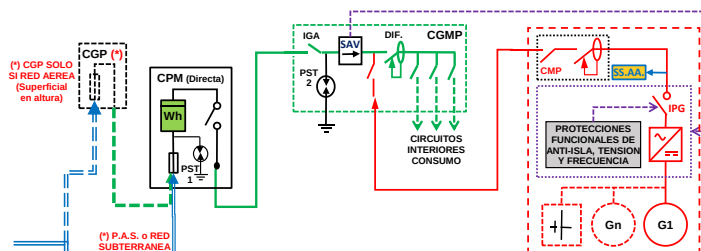
ESQUEMA 1 Individual - SIN Excedentes - en CGMP Red interior - Generación (Ren-Co-Res y mismo Titular) - Finca 1 Suministro - PgII = Cualquiera - PCG ≤ 50 kW - Modo Dependiente
