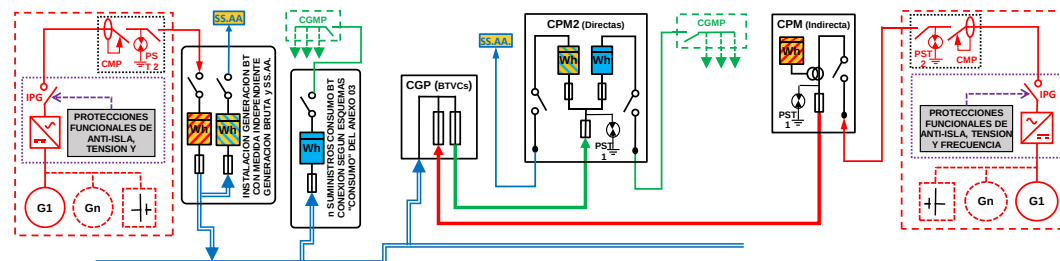
ESQUEMA 148 (Opcional a ESQUEMA 141 con medida en paralelo de Generación Bruta, SS.AA. y Consumo) Colectivo - CON Venta Excedentes - Mixta: a través Red Distribución y en Instalación Enlace - Finca 1 Suministro - 50 < PglE ≤ 100 kW - Pc ≤ 400 kW - Modo Dependiente
