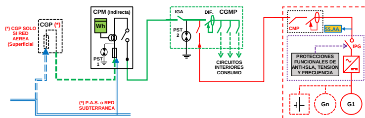
ESQUEMA 16 Individual - CON Compensación Excedentes - en CGMP Red interior - Generación (Renovable y mismo titular) - Finca 1 Suministro - 50 < P_{gII} \leq 100 \text{ kW} ó 50 < P_{CG} \leq 400 \text{ kW} - Modo Dependiente
