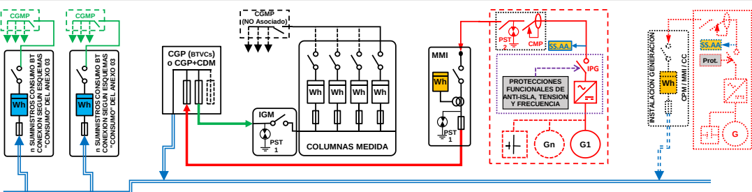
ESQUEMA 124 Colectivo - CON Venta Excedentes - A través Red Distribución - Finca \geq 2 Suministros - 50 < P_{gIE} \leq 100 \text{ kW} - P_c \leq 400 \text{ kW} - Modo Dependiente
