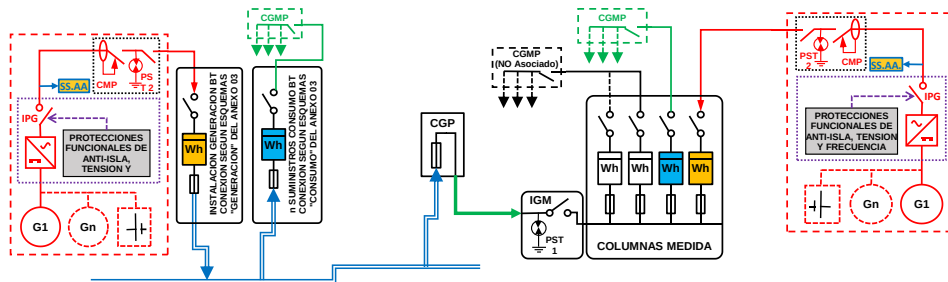
ESQUEMA 142 (Opcional a ESQUEMAS 134 ó 135 con medida en paralelo de Generación Neta y Consumo) Colectivo - CON Venta Excedentes - Mixta: a través Red Distribución y en Instalación Enlace - Finca \geq 2 Suministros - P_{glE} \leq 50 kW - P_c \leq 50 kW - Modo Dependiente
