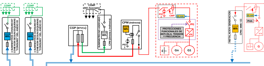
ESQUEMA 122 Colectivo - CON Venta Excedentes - A través Red Distribución - Finca 1 Suministro - 50 < P_{gIE} \leq 100 \text{ kW} - P_c \leq 400 \text{ kW} - Modo Dependiente
