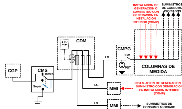
FIGURA M57 - CONMUTACION MODO SEPARADO EN AUTOCONSUMOS COLECTIVOS CON GENERACION EN CC o MMI
