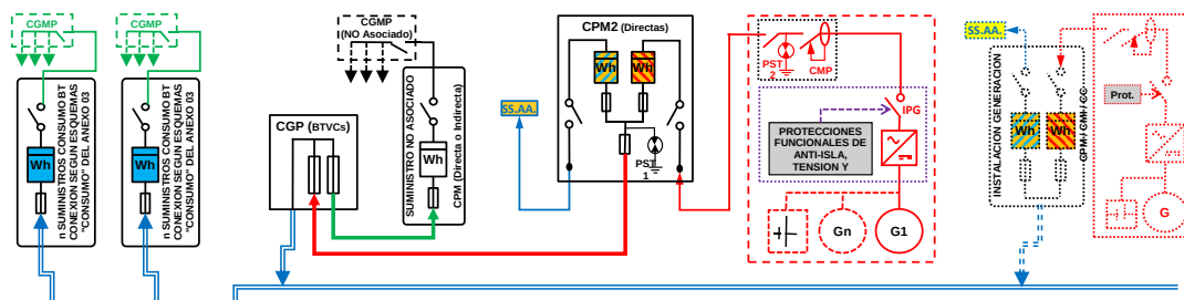
ESQUEMA 127 (Opcional a ESQUEMA 121 con medida en paralelo de Generación Bruta, SS.AA. y Consumo) Colectivo - CON Venta Excedentes - A través Red Distribución - Finca 1 Suministro - P_{gIE} \leq 50 \text{ kW} - P_c \leq 400 \text{ kW} - Modo Dependiente
