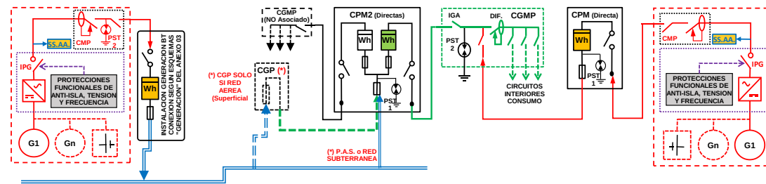
ESQUEMA 58 Individual - CON Venta Excedentes - Mixta: a través Red Distribución y en CGMP Red interior - Finca 2 Suministros - PglI ≤ 50 kW - PCG ≤ 50 kW - Modo Dependiente
