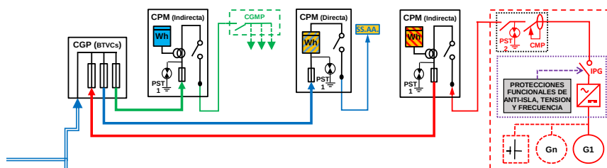
ESQUEMA 38 (Opcional a ESQUEMA 30 con medida en paralelo de Generación Bruta, SS.AA. y Consumo) Individual - CON Venta Excedentes - en Instalación Enlace Red interior - Finca 1 Suministro - 50 < P_{glE} \leq 100 \text{ kW} - 50 < P_c \leq 400 \text{ kW} - Modo Dependiente
