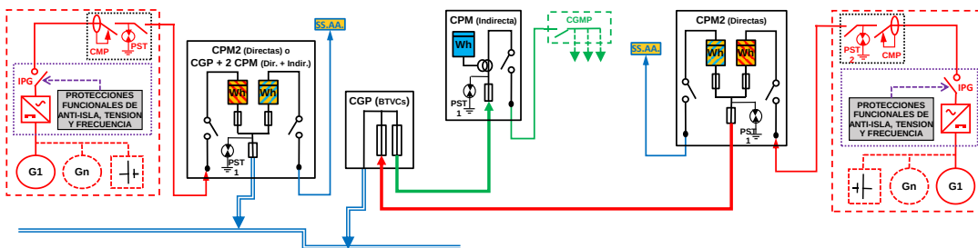
ESQUEMA 72 (Opcional a ESQUEMA 64 con medida en paralelo de Generación Bruta, SS.AA. y Consumo) Individual - CON Venta Excedentes - Mixta: a través Red Distribución y en Instalación Enlace - Finca 1 Suministro - 50 < P_{glE} \leq 100 \text{ kW} - P_c \leq 50 \text{ kW} - Modo Dependiente
