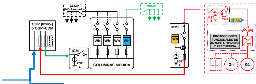
ESQUEMA 33 (Opcional a ESQUEMAS 19 (Si 50 < P_{gIE} \leq 100 kW) y 26 (Si P_c \leq 50 kW) con medida en paralelo de Generación Neta y Consumo) Individual - CON Venta Excedentes - en Instalación Enlace Red interior - Finca \geq 2 Suministros - 50 < P_{gIE} \leq 100 kW - P_c \leq 50 kW - Modo Dependiente
