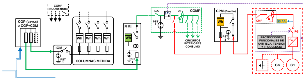
ESQUEMA 13 Individual - SIN Excedentes - en CGMP Red interior - Generación (NO Ren-Co-Res o Distinto Titular o Hibridación) - Finca \geq 2 Suministros - 50 < P_{gII} \leq 250 kW - PCG \leq 250 kW - Modo Dependiente
