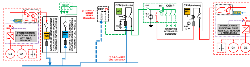
ESQUEMA 134 Colectivo - CON Venta Excedentes - Mixta: a través Red Distribución y en CGMP Red interior - Finca 2 Suministros - P_{glt} \leq 50 kW - PCG \leq 50 kW - Modo Dependiente
