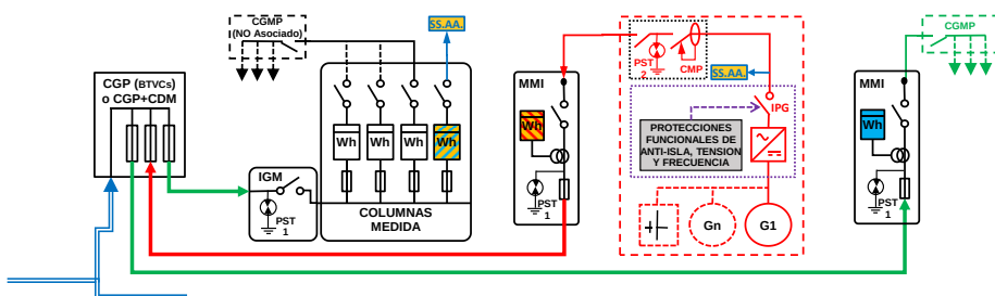
ESQUEMA 42 (Opcional a ESQUEMA 34 con medida en paralelo de Generación Bruta, SS.AA. y Consumo) Individual - CON Venta Excedentes - en Instalación Enlace Red interior - Cualquier Finca - 50 < P_{gIE} \leq 100 \text{ kW} - 50 < P_c \leq 250 \text{ kW} - Modo Dependiente
