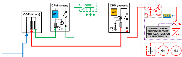
ESQUEMA 29 (Opcional a ESQUEMAS 16 (Si 50 < P_{gII} \leq 100 kW) y 22 (Si P_c \leq 50 kW) con medida en paralelo de Generación Neta y Consumo) Individual - CON Venta Excedentes - en Instalación Enlace Red interior - Finca 1 Suministro - 50 < P_{gIE} \leq 100 kW - P_c \leq 50 kW - Modo Dependiente
