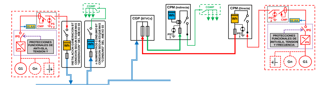
ESQUEMA 140 (Opcional a ESQUEMA 133 (Si PCG \leq 50 \text{ kW} ) con medida en paralelo de Generación Neta y Consumo) Colectivo - CON Venta Excedentes - Mixta: a través Red Distribución y en Instalación Enlace - Finca 1 Suministro - 50 < P_{gIE} \leq 100 \text{ kW} - P_c \leq 50 \text{ kW} - Modo Dependiente
