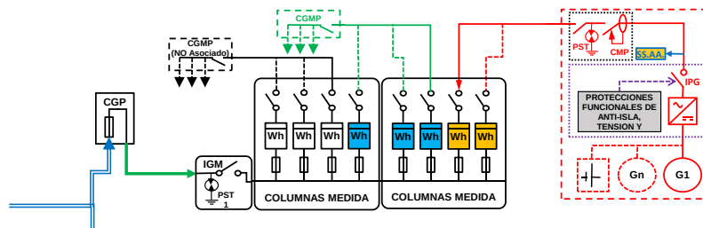
ESQUEMA 93 (Opcional a ESQUEMA 90 con medida en paralelo de Generación Neta y Consumo) Colectivo - CON compensación (si Renovable) o Venta Excedentes - en Instalación Enlace Red interior - Finca \geq 2 Suministros - P_{gIE} \leq 50 kW - P_c \leq 250 kW - Modo Dependiente
