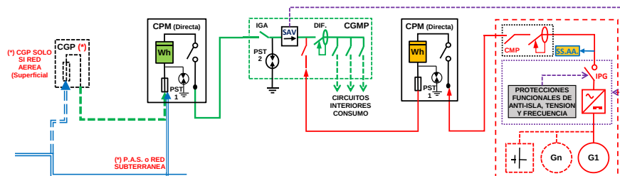
ESQUEMA 6 Individual - SIN Excedentes - en CGMP Red interior - Generación (NO Ren-Co-Res o Distinto Titular o Hibridación) - Finca 1 Suministro - P_{gII} \leq 50 \text{ kW} - PCG \leq 50 \text{ kW} - Modo
