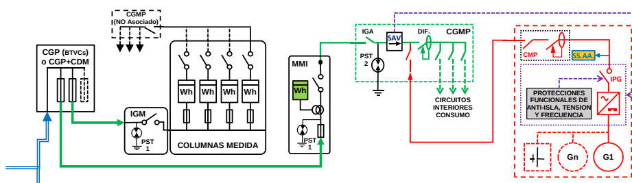
ESQUEMA 5 Individual - SIN Excedentes - en CGMP Red interior - Generación (Ren-Co-Res y mismo Titular) - Finca ≥ 2 Suministros - PgII = Cualquiera - 50 < PCG ≤ 250 kW - Modo
