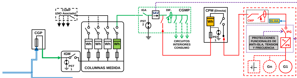
ESQUEMA 12 Individual - SIN Excedentes - en CGMP Red interior - Generación (NO Ren-Co-Res o Distinto Titular o Hibridación) - Finca \geq 2 Suministros - P_{gII} \leq 50 kW - 50 < PCG \leq 250 kW - Modo Dependiente
