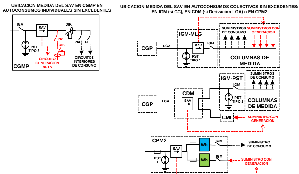
Figura 2. Ubicación preferente de la medida del SAV.
