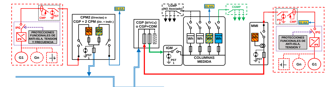
ESQUEMA 76 (Opcional a ESQUEMA 68 con medida en paralelo de Generación Bruta, SS.AA. y Consumo) Individual - CON Venta Excedentes - Mixta: a través Red Distribución y en Instalación Enlace - Finca \geq 2 Suministros - 50 < P_{gIE} \leq 100 kW - P_c \leq 50 kW - Modo Dependiente
