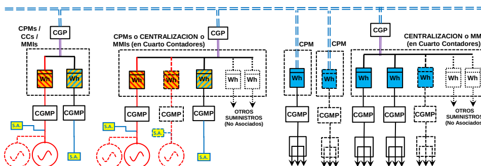
ESQUEMA MEDIDA "D (CR)" (Colectivo a través de Red de distribución) (1 Contador bidireccional en Frontera de cada consumidor + 1 contador en cada Generación Bruta + 1 contador en cada SS.AA.)
