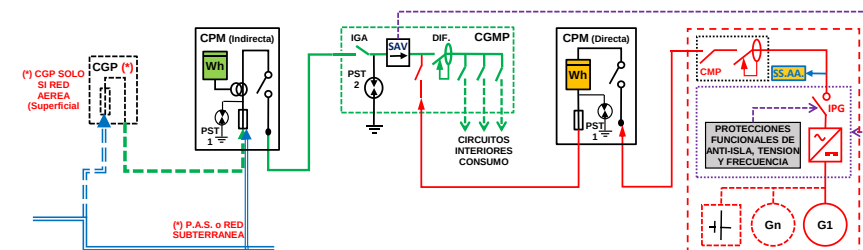
ESQUEMA 7 Individual - SIN Excedentes - en CGMP Red interior - Generación (NO Ren-Co-Res o Distinto Titular o Hibridación) - Finca 1 Suministro - P_{gII} \leq 50 \text{ kW} - 50 < PCG \leq 400 \text{ kW} - Modo
