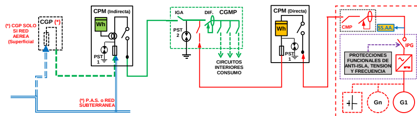
ESQUEMA 21 Individual - CON Venta Excedentes - en CGMP Red interior - Generación (NO Ren-Co-Res o Distinto Titular o Hibridación) - Finca 1 Suministro - P_{gII} \leq 50 \text{ kW} - 50 < PCG \leq 400 \text{ kW} - Modo Dependiente
