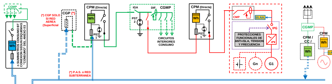
ESQUEMA 98 Colectivo - CON compensación (si Renovable) o Venta Excedentes - Compartida: a través Red Distribución y 100% generación en CGMP instalación interior - Finca 1 Suministro - P_{gII} \leq 50 kW - PCG \leq 50 kW - Modo Dependiente
