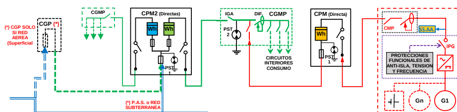
ESQUEMA 88 Colectivo - CON compensación (si Renovable) o Venta Excedentes - en CGMP Red interior - Finca 2 Suministros - P_{gII} \leq 50 kW - PCG \leq 50 kW - Modo Dependiente
