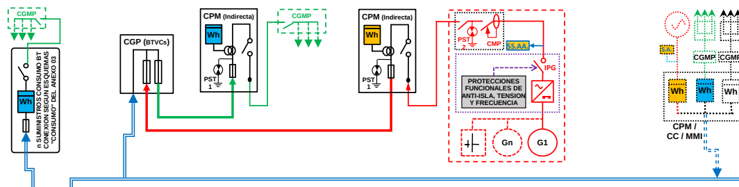
ESQUEMA 109 (Opcional a ESQUEMA 101 ó 102 con medida en paralelo de Generación Neta y Consumo) Colectivo - CON compensación (si Renovable) o Venta Excedentes - Compartida: a través Red Distribución y 100% generación en instalación enlace edificio - Finca \geq 2 Suministros - P_{gIE} \leq 50 \text{ kW} - P_c \leq 50 \text{ kW} - Modo Dependiente
