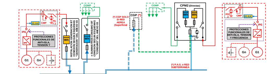
ESQUEMA 139 (Opcional a ESQUEMA 132 con medida en paralelo de Generación Neta y Consumo) Colectivo - CON Venta Excedentes - Mixta: a través Red Distribución y en Instalación Enlace - Finca 1 Suministro - P_{gIE} \leq 50 \text{ kW} - P_c \leq 400 \text{ kW} - Modo Dependiente
