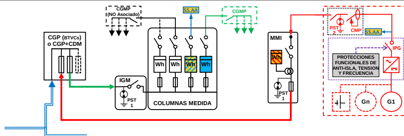
ESQUEMA 41 (Opcional a ESQUEMA 33 con medida en paralelo de Generación Bruta, SS.AA. y Consumo) Individual - CON Venta Excedentes - en Instalación Enlace Red interior - Cualquier Finca - 50 < P_{gIE} \leq 100 \text{ kW} - P_c \leq 50 \text{ kW} - Modo Dependiente
