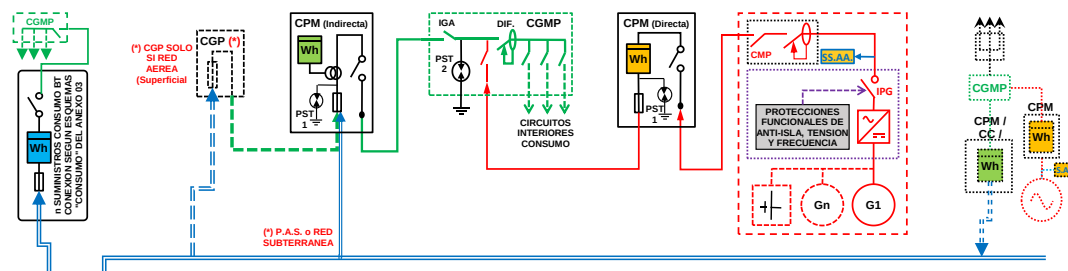
ESQUEMA 99 Colectivo - CON compensación (si Renovable) o Venta Excedentes - Compartida: a través Red Distribución y 100% generación en CGMP instalación interior - Finca 1 Suministro - P_{gII} \leq 50 kW - 50 < PCG \leq 400 kW - Modo Dependiente
