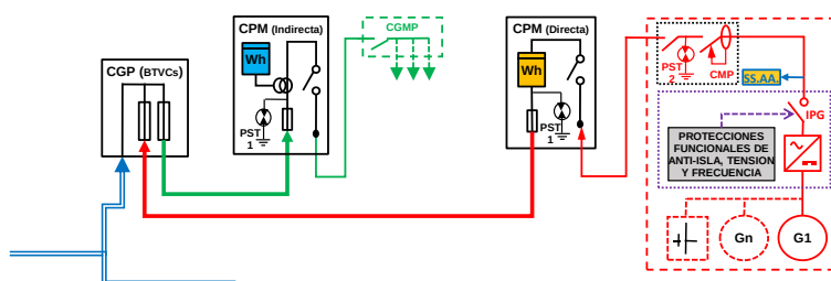
ESQUEMA 28 (Opcional a ESQUEMAS 16 (Si P_{gII} \leq 50 kW) y 21 con medida en paralelo de Generación Neta y Consumo) Individual - CON Venta Excedentes - en Instalación Enlace Red interior - Finca 1 Suministro - P_{gIE} \leq 50 kW - 50 < P_c \leq 400 kW - Modo Dependiente
