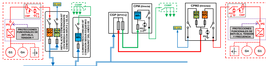
ESQUEMA 145 (Opcional a ESQUEMA 138 con medida en paralelo de Generación Bruta, SS.AA. y Consumo) Colectivo - CON Venta Excedentes - Mixta: a través Red Distribución y en Instalación Enlace - Finca 1 Suministro - P_{glE} \leq 50 kW - P_c \leq 50 kW - Modo Dependiente
