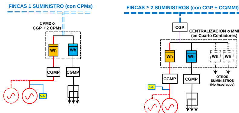
ESQUEMA MEDIDA "C (II)" (Individual en red Interior: en "Paralelo" en instalación de enlace) (1 Contador en Consumo Total + 1 contador bidireccional en Generación Neta)
