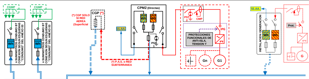
ESQUEMA 125 (Opcional a ESQUEMA 119 con medida en paralelo de Generación Bruta, SS.AA. y Consumo) Colectivo - CON Venta Excedentes - A través Red Distribución - Conexión directa a red - P_{gRD} \leq 50 \text{ kW} - P_c \leq 400 \text{ kW} - Modo Dependiente
