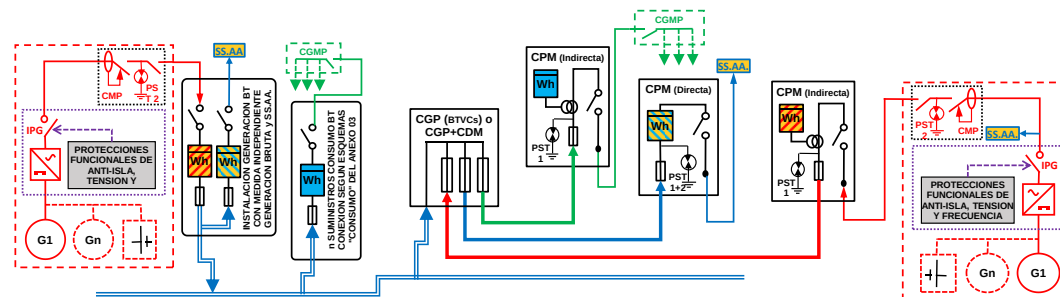
ESQUEMA 149 (Opcional a ESQUEMAS 142 con medida en paralelo de Generación Bruta, SS.AA. y Consumo) Colectivo - CON Venta Excedentes - Mixta: a través Red Distribución y en Instalación Enlace - Finca ≥ 2 Suministros - PglE ≤ 50 kW - Pc ≤ 50 kW - Modo Dependiente
