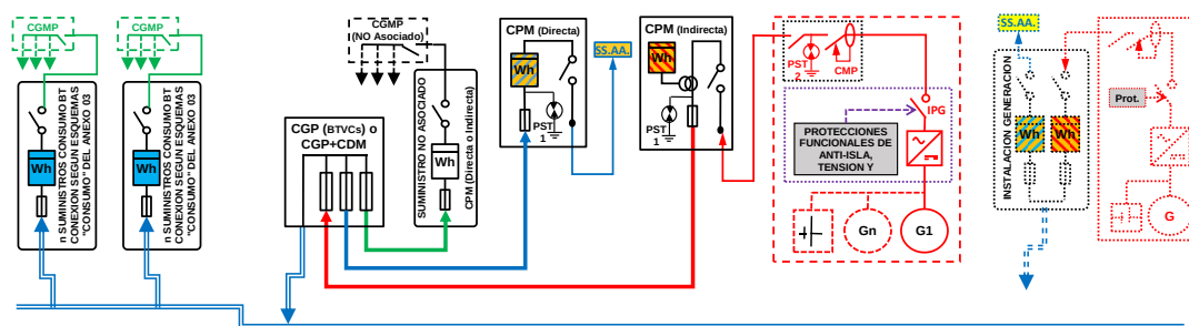
ESQUEMA 129 (Opcional a ESQUEMA 123 con medida en paralelo de Generación Bruta, SS.AA. y Consumo) Colectivo - CON Venta Excedentes - A través Red Distribución - Finca \geq 2 Suministros - P_{gIE} \leq 50 \text{ kW} - P_c \leq 400 \text{ kW} - Modo Dependiente
