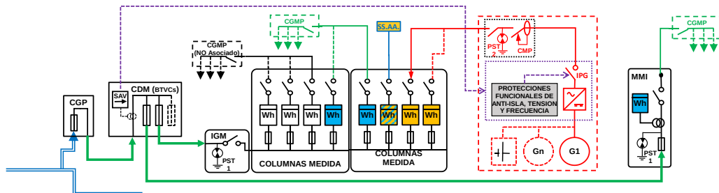
ESQUEMA 86 (Opcional a ESQUEMA 83 con medida en paralelo de Generación Bruta, SS.AA. y Consumo) Colectivo - SIN Excedentes - en Instalación Enlace Red interior - Finca \geq 2 Suministros - P_{gIE} \leq 50 kW - P_c \leq 250 kW - Modo Dependiente
