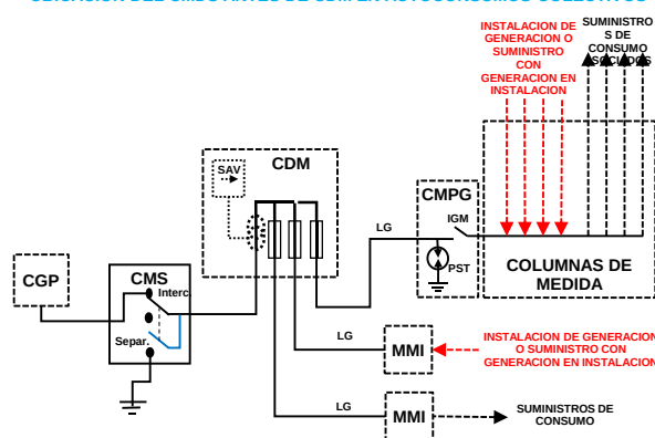
UBICACION DEL CMDS ANTES DE CDM EN AUTOCONSUMOS COLECTIVOS
