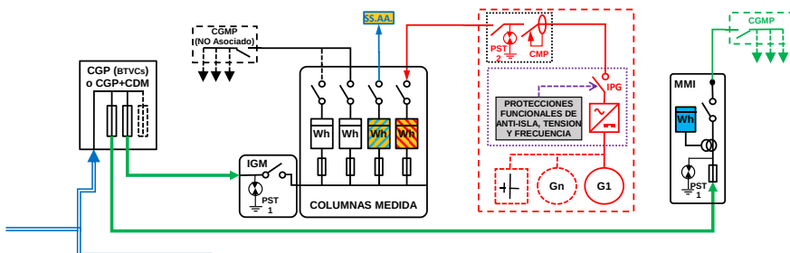
ESQUEMA 40 (Opcional a ESQUEMA 32 con medida en paralelo de Generación Bruta, SS.AA. y Consumo) Individual - CON Venta Excedentes - en Instalación Enlace Red interior - Cualquier Finca - Pg/E ≤ 50 kW - 50 < Pc ≤ 250 kW - Modo Dependiente
