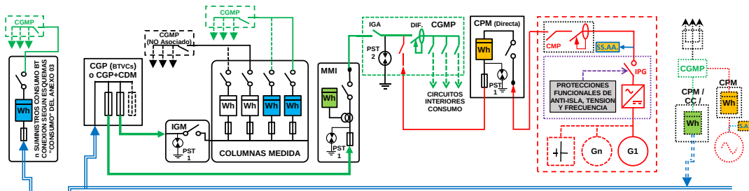
ESQUEMA 103 Colectivo - CON compensación (si Renovable) o Venta Excedentes - Compartida: a través Red Distribución y 100% generación en CGMP instalación interior - Finca \geq 2 Suministros - P_{gII} \leq 50 \text{ kW} - 50 < PCG \leq 250 \text{ kW} - Modo Dependiente
