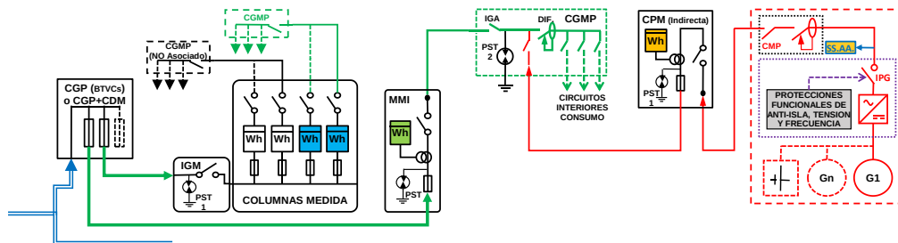
ESQUEMA 92 (Opcional a ESQUEMA 88 ó 89 con medida en paralelo de Generación Neta y Consumo) Colectivo - CON compensación (si Renovable) o Venta Excedentes - en Instalación Enlace Red interior - Finca \geq 2 Suministros - P_{gIE} \leq 50 kW - P_c \leq 50 kW - Modo Dependiente
