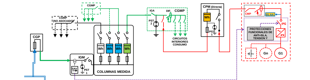
ESQUEMA 79 Colectivo - SIN Excedentes - en CGMP Red interior - Finca \geq 2 Suministros - P_{gII} \leq 50 kW - PCG \leq 50 kW - Modo Dependiente
