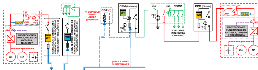
ESQUEMA 133 Colectivo - CON Venta Excedentes - Mixta: a través Red Distribución y en CGMP Red interior - Finca 1 Suministro - 50 < P_{glt} \leq 100 kW - PCG \leq 400 kW - Modo Dependiente
