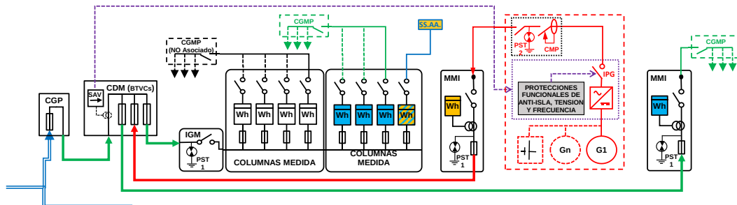
ESQUEMA 87 (Opcional a ESQUEMA 84 con medida en paralelo de Generación Bruta, SS.AA. y Consumo) Colectivo - SIN Excedentes - en Instalación Enlace Red interior - Finca \geq 2 Suministros - 50 < P_{gIE} \leq 250 kW - P_c \leq 250 kW - Modo Dependiente
