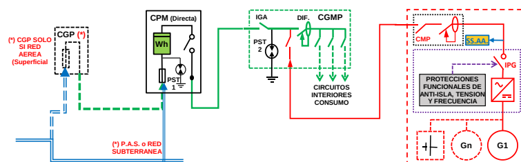
ESQUEMA 15 Individual - CON Compensación Excedentes - en CGMP Red interior - Generación (Renovable y mismo titular) - Finca 1 Suministro - P_{gII} \leq 50 kW - PCG \leq 50 kW - Modo Dependiente
