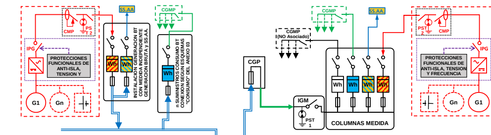
ESQUEMA 150 (Opcional a ESQUEMAS 143 con medida en paralelo de Generación Bruta, SS.AA. y Consumo) Colectivo - CON Venta Excedentes - Mixta: a través Red Distribución y en Instalación Enlace - Finca ≥ 2 Suministros - PglE ≤ 50 kW - Pc ≤ 250 kW - Modo Dependiente
