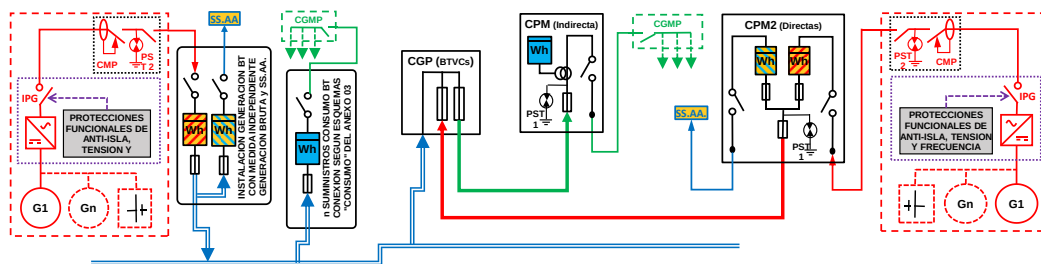
ESQUEMA 147 (Opcional a ESQUEMA 140 con medida en paralelo de Generación Bruta, SS.AA. y Consumo) Colectivo - CON Venta Excedentes - Mixta: a través Red Distribución y en Instalación Enlace - Finca 1 Suministro - 50 < PglE ≤ 100 kW - Pc ≤ 50 kW - Modo Dependiente
