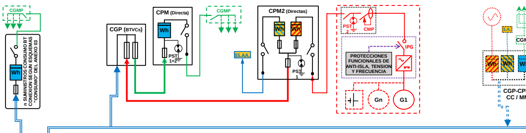
ESQUEMA 112 (Opcional a ESQUEMA 105 con medida en paralelo de Generación Bruta, SS.AA. y Consumo) Colectivo - CON compensación (si Renovable) o Venta Excedentes - Compartida: a través Red Distribución y 100% generación en instalación enlace edificio - Finca 1 Suministro - P_{gIE} \leq 50 kW - P_c \leq 50 kW - Modo Dependiente
