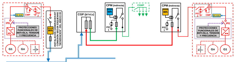
ESQUEMA 65 (Opcional a ESQUEMA 57 (Si 50 < PCG \leq 400 kW) con medida en paralelo de Generación Neta y Consumo) Individual - CON Venta Excedentes - Mixta: a través Red Distribución y en Instalación Enlace - Finca 1 Suministro - 50 < P_{gIE} \leq 100 kW - P_c \leq 400 kW - Modo Dependiente
