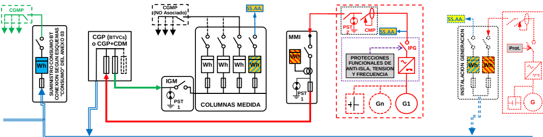
ESQUEMA 54 (Opcional a ESQUEMA 48 con medida en paralelo de Generación Bruta, SS.AA. y Consumo) Individual - CON Venta Excedentes - A través Red Distribución - Finca ≥ 2 Suministros - 50 < PgRD ≤ 100 kW - Pc ≤ 400 kW - Modo Dependiente
