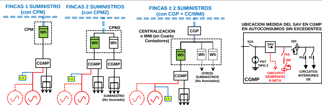
ESQUEMA MEDIDA "A" (Genérica: Individual en CGMP de instalación interior) (1 Contador bidireccional en Frontera del Consumidor)
