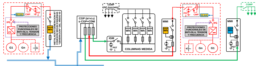
ESQUEMA 69 (Opcional a ESQUEMA 61 (Si 50 < PCG \leq 250 kW) con medida en paralelo de Generación Neta y Consumo) Individual - CON Venta Excedentes - Mixta: a través Red Distribución y en Instalación Enlace - Finca \geq 2 Suministros - 50 < P_{gIE} \leq 100 kW - 50 < P_c \leq 250 kW - Modo Dependiente
