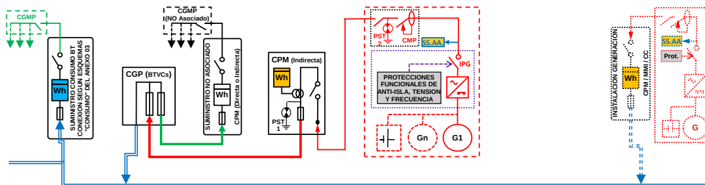
ESQUEMA 47 Individual - CON Venta Excedentes - A través Red Distribución - Finca \geq 2 Suministros - PgRD \leq 50 kW - P_c \leq 400 kW - Modo Dependiente
