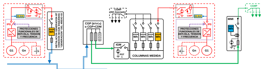
ESQUEMA 67 (Opcional a ESQUEMA 60 con medida en paralelo de Generación Neta y Consumo) Individual - CON Venta Excedentes - Mixta: a través Red Distribución y en Instalación Enlace - Finca \geq 2 Suministros - P_{gIE} \leq 50 kW - 50 < P_c \leq 250 kW - Modo Dependiente
