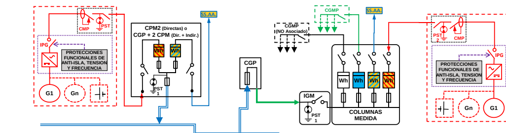
ESQUEMA 75 (Opcional a ESQUEMA 67 con medida en paralelo de Generación Bruta, SS.AA. y Consumo) Individual - CON Venta Excedentes - Mixta: a través Red Distribución y en Instalación Enlace - Finca \geq 2 Suministros - P_{glE} \leq 50 \text{ kW} - 50 < P_c \leq 250 \text{ kW} - Modo Dependiente
