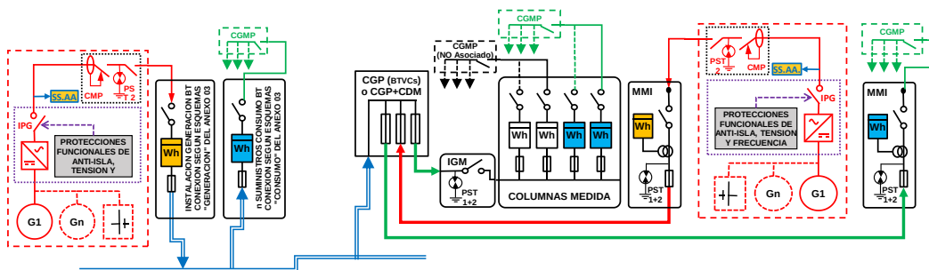
ESQUEMA 145 (Opcional a ESQUEMA 138 con medida en paralelo de Generación Bruta, SS.AA. y Consumo) Colectivo - CON Venta Excedentes - Mixta: a través Red Distribución y en Instalación Enlace - Finca 1 Suministro - P_{glE} \leq 50 kW - P_c \leq 50 kW - Modo Dependiente
