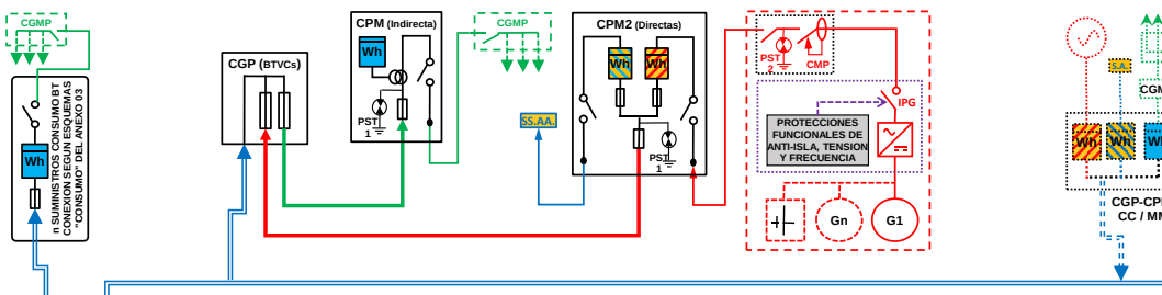
ESQUEMA 114 (Opcional a ESQUEMA 107 con medida en paralelo de Generación Bruta, SS.AA. y Consumo) Colectivo - CON compensación (si Renovable) o Venta Excedentes - Compartida: a través Red Distribución y 100% generación en instalación enlace edificio - Finca 1 Suministro - 50 < P_{gIE} \leq 100 kW - P_c \leq 50 kW - Modo Dependiente
