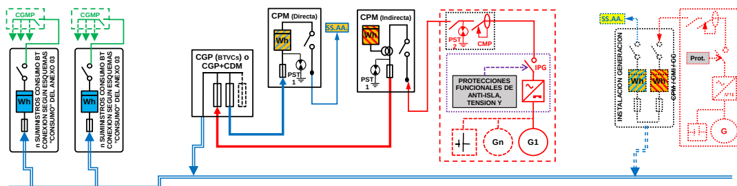
ESQUEMA 126 (Opcional a ESQUEMA 120 con medida en paralelo de Generación Bruta, SS.AA. y Consumo) Colectivo - CON Venta Excedentes - A través Red Distribución - Conexión directa a red - 50 < P_{gRD} \leq 100 \text{ kW} - P_c \leq 400 \text{ kW} - Modo Dependiente
