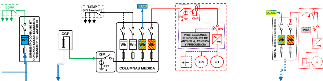
ESQUEMA 53 (Opcional a ESQUEMA 47 con medida en paralelo de Generación Bruta, SS.AA. y Consumo) Individual - CON Venta Excedentes - A través Red Distribución - Finca ≥ 2 Suministros - PgRD ≤ 50 kW - Pc ≤ 400 kW - Modo Dependiente
