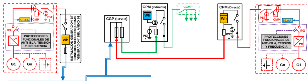
ESQUEMA 63 (Opcional a ESQUEMA 56 con medida en paralelo de Generación Neta y Consumo) Individual - CON Venta Excedentes - Mixta: a través Red Distribución y en Instalación Enlace - Finca 1 Suministro - P_{gIE} \leq 50 kW - P_c \leq 400 kW - Modo Dependiente
