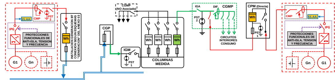
ESQUEMA 59 Individual - CON Venta Excedentes - Mixta: a través Red Distribución y en CGMP Red interior - Finca ≥ 2 Suministros - PglI ≤ 50 kW - PCG ≤ 50 kW - Modo Dependiente
