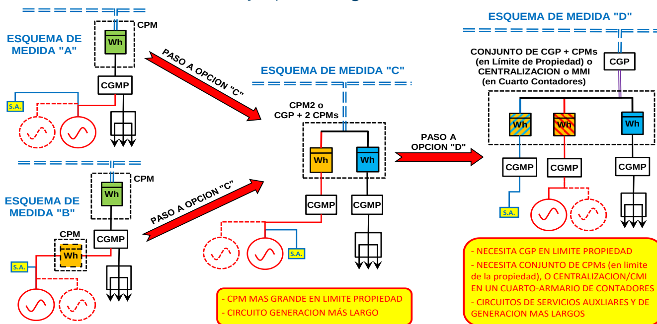
Figura 1. Implicaciones de optar por esquemas de medida C o D.
