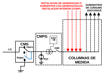
FIGURA M57 - CONMUTACION MODO SEPARADO EN AUTOCONSUMOS COLECTIVOS CON GENERACION EN CC o MMI
