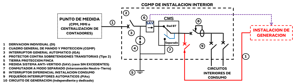
FIGURA MS2 - CONMUTACION MODO SEPARADO EN AUTOCONSUMO INDIVIDUAL CON EXCEDENTES CON GENERACION CONECTADA EN CGMP INSTALACION INTERIOR
