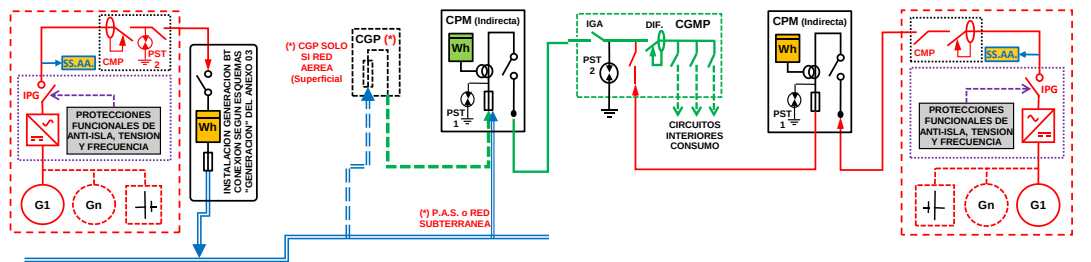
ESQUEMA 57 Individual - CON Venta Excedentes - Mixta: a través Red Distribución y en CGMP Red interior - Finca 1 Suministro - 50 < PglI ≤ 100 kW - PCG ≤ 400 kW - Modo Dependiente
