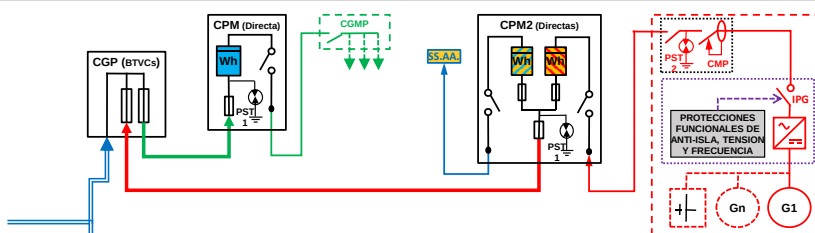
ESQUEMA 35 (Opcional a ESQUEMA 27 con medida en paralelo de Generación Bruta, SS.AA. y Consumo) Individual - CON Venta Excedentes - en Instalación Enlace Red interior - Finca 1 Suministro - P_{gIE} \leq 50 kW - P_c \leq 50 kW - Modo Dependiente
