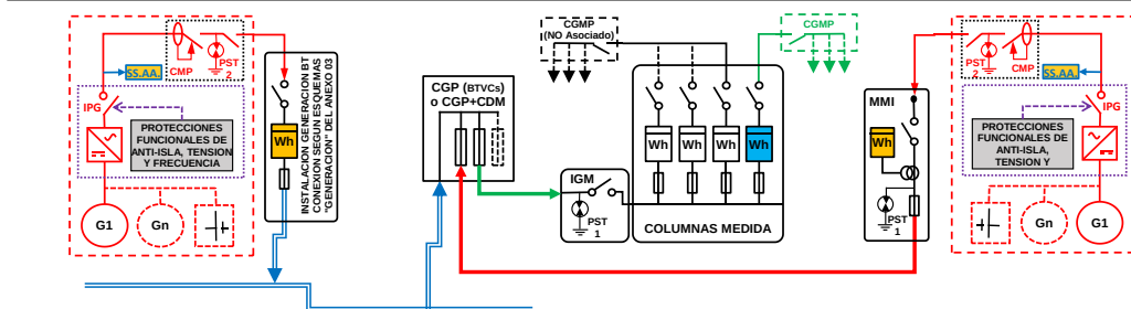
ESQUEMA 69 (Opcional a ESQUEMA 61 (Si 50 < PCG \leq 250 kW) con medida en paralelo de Generación Neta y Consumo) Individual - CON Venta Excedentes - Mixta: a través Red Distribución y en Instalación Enlace - Finca \geq 2 Suministros - 50 < P_{gIE} \leq 100 kW - 50 < P_c \leq 250 kW - Modo Dependiente
