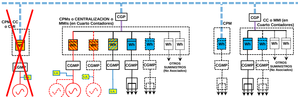
ESQUEMA MEDIDA "D (CC)" (Colectivo Compartido: a través red y en "Paralelo" en instalación enlace) (1 Contador bidireccional en Frontera de cada consumidor + 1 contador en cada Generación Bruta + 1 contador en cada SS.AA.)
