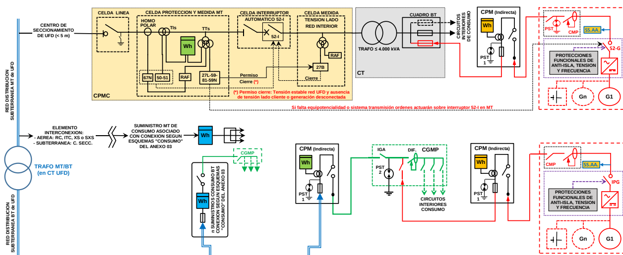
Figura 6. Ejemplo 2 Autoconsumo Combinado (AT/BT).
