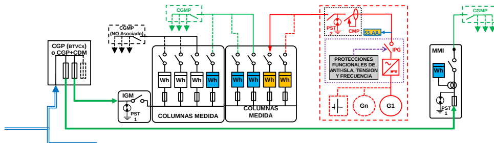
ESQUEMA 93 (Opcional a ESQUEMA 90 con medida en paralelo de Generación Neta y Consumo) Colectivo - CON compensación (si Renovable) o Venta Excedentes - en Instalación Enlace Red interior - Finca \geq 2 Suministros - P_{gIE} \leq 50 kW - P_c \leq 250 kW - Modo Dependiente
