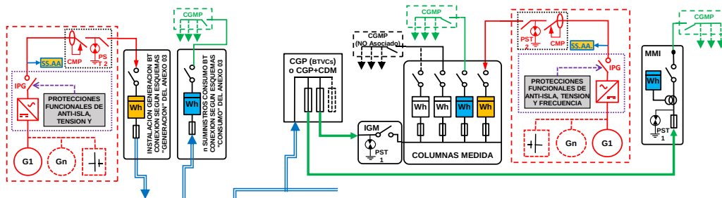
ESQUEMA 144 (Opcional a ESQUEMA 137 con medida en paralelo de Generación Neta y Consumo) Colectivo - CON Venta Excedentes - Mixta: a través Red Distribución y en Instalación Enlace - Finca \geq 2 Suministros - 50 < P_{glE} \leq 100 kW - P_c \leq 250 kW - Modo Dependiente
