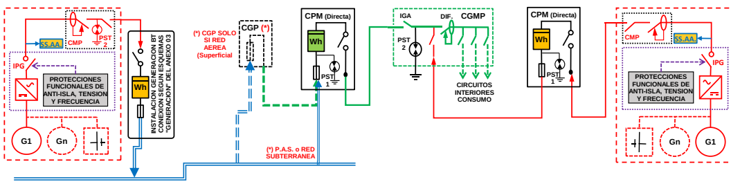
ESQUEMA 55 Individual - CON Venta Excedentes - Mixta: a través Red Distribución y en CGMP Red interior - Finca 1 Suministro - Pgll ≤ 50 kW - PCG ≤ 50 kW - Modo Dependiente
