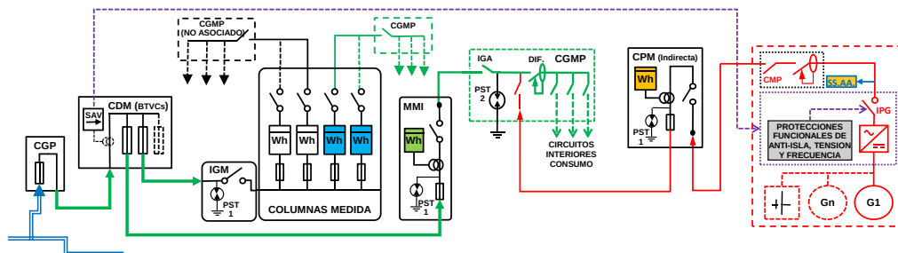
ESQUEMA 81 Colectivo - SIN Excedentes - en CGMP Red interior - Finca \geq 2 Suministros - 50 < P_{gII} \leq 250 kW - PCG \leq 250 kW - Modo Dependiente
