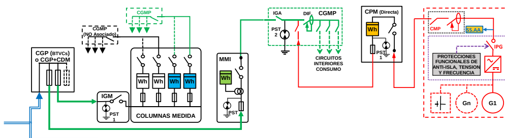
ESQUEMA 90 Colectivo - CON compensación (si Renovable) o Venta Excedentes - en CGMP Red interior - Finca \geq 2 Suministros - P_{gII} \leq 50 kW - 50 < PCG \leq 250 kW - Modo Dependiente
