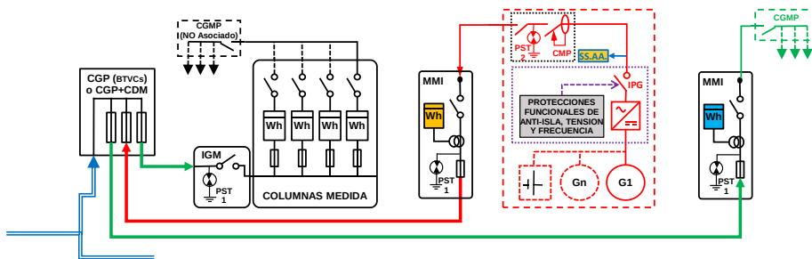
ESQUEMA 34 (Opcional a ESQUEMAS 19 (Si 50 < P_{gIE} \leq 100 kW) y 26 (Si 50 < P_c \leq 250 kW) con medida en paralelo de Generación Neta y Consumo) Individual - CON Venta Excedentes - en Instalación Enlace Red interior - Finca \geq 2 Suministros - 50 < P_{gIE} \leq 100 kW - 50 < P_c \leq 250 kW - Modo Dependiente
