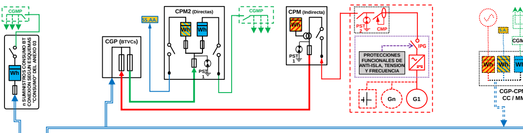
ESQUEMA 115 (Opcional a ESQUEMA 108 con medida en paralelo de Generación Bruta, SS.AA. y Consumo) Colectivo - CON compensación (si Renovable) o Venta Excedentes - Compartida: a través Red Distribución y 100% generación en instalación enlace edificio - Finca 1 Suministro - 50 < P_{gIE} \leq 100 kW - P_c \leq 400 kW - Modo Dependiente
