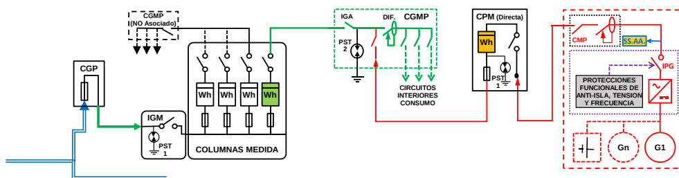
ESQUEMA 24 Individual - CON Venta Excedentes - en CGMP Red interior - Generación (NO Ren-Co-Res o Distinto Titular o Hibridación) - Finca \geq 2 Suministros - P_{gII} \leq 50 \text{ kW} - PCG \leq 50 \text{ kW} - Modo Dependiente
