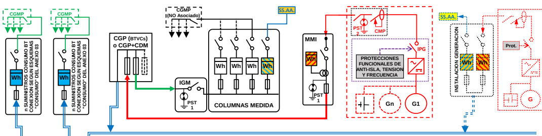
ESQUEMA 130 (Opcional a ESQUEMA 124 con medida en paralelo de Generación Bruta, SS.AA. y Consumo) Colectivo - CON Venta Excedentes - A través Red Distribución - Finca \geq 2 Suministros - 50 < P_{gIE} \leq 100 \text{ kW} - P_c \leq 400 \text{ kW} - Modo Dependiente
