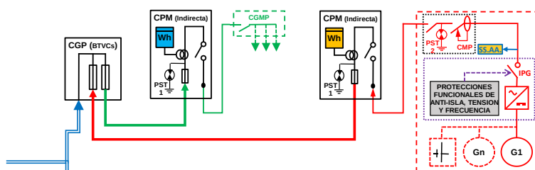
ESQUEMA 30 (Opcional a ESQUEMAS 16 (Si 50 < P_{gII} \leq 100 kW) y 22 (Si 50 < P_c \leq 400 kW) con medida en paralelo de Generación Neta y Consumo) Individual - CON Venta Excedentes - en Instalación Enlace Red interior - Finca 1 Suministro - 50 < P_{gIE} \leq 100 kW - 50 < P_c \leq 400 kW - Modo Dependiente
