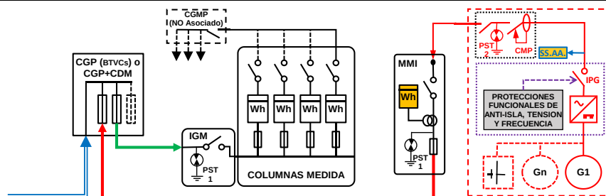
ESQUEMA MEDIDA "A" (Genérica: Individual en CGMP de instalación interior) (1 Contador bidireccional en Frontera del Consumidor)
