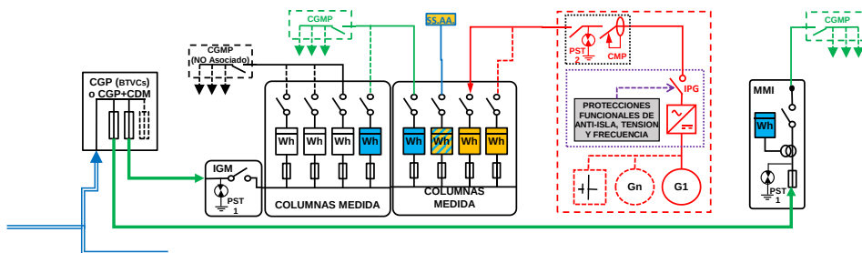
ESQUEMA 97 (Opcional a ESQUEMA 94 con medida en paralelo de Generación Bruta, SS.AA. y Consumo) Colectivo - CON compensación (si Renovable) o Venta Excedentes - en Instalación Enlace Red interior - Finca \geq 2 Suministros - 50 < P_{gIE} \leq 100 kW - P_c \leq 250 kW - Modo Dependiente
