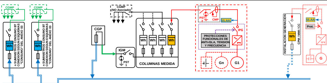
ESQUEMA 123 Colectivo - CON Venta Excedentes - A través Red Distribución - Finca \geq 2 Suministros - P_{gIE} \leq 50 \text{ kW} - P_c \leq 400 \text{ kW} - Modo Dependiente
