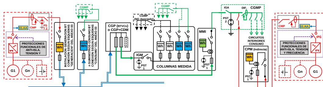
ESQUEMA 138 (Opcional a ESQUEMA 131 con medida en paralelo de Generación Neta y Consumo) Colectivo - CON Venta Excedentes - Mixta: a través Red Distribución y en Instalación Enlace - Finca 1 Suministro - P_{gIE} \leq 50 \text{ kW} - P_c \leq 50 \text{ kW} - Modo Dependiente
