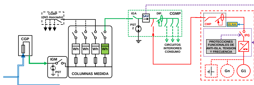
ESQUEMA 4 Individual - SIN Excedentes - en CGMP Red interior - Generación (Ren-Co-Res y mismo Titular) - Finca ≥ 2 Suministros - PgII = Cualquiera - PCG ≤ 50 kW - Modo Dependiente
