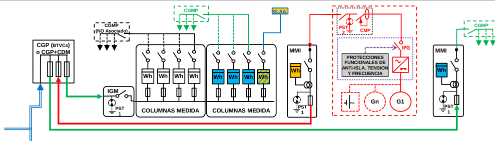
ESQUEMA 98 Colectivo - CON compensación (si Renovable) o Venta Excedentes - Compartida: a través Red Distribución y 100% generación en CGMP instalación interior - Finca 1 Suministro - P_{gII} \leq 50 kW - PCG \leq 50 kW - Modo Dependiente
