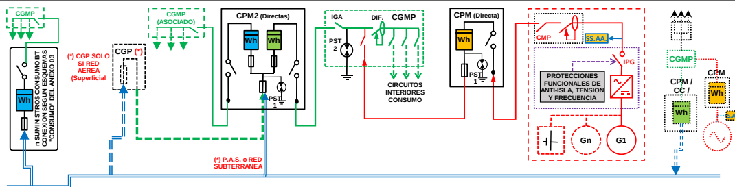
ESQUEMA 102 Colectivo - CON compensación (si Renovable) o Venta Excedentes - Compartida: a través Red Distribución y 100% generación en CGMP instalación interior - Finca \geq 2 Suministros - P_{gII} \leq 50 \text{ kW} - PCG \leq 50 \text{ kW} - Modo Dependiente
