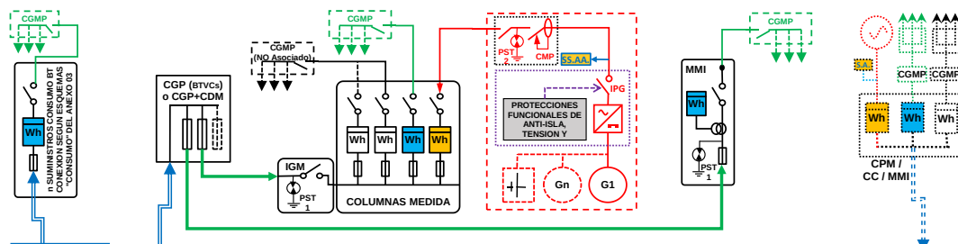
ESQUEMA 110 (Opcional a ESQUEMA 103 con medida en paralelo de Generación Neta y Consumo) Colectivo - CON compensación (si Renovable) o Venta Excedentes - Compartida: a través Red Distribución y 100% generación en instalación enlace edificio - Finca \geq 2 Suministros - P_{gIE} \leq 50 \text{ kW} - P_c \leq 250 \text{ kW} - Modo Dependiente
