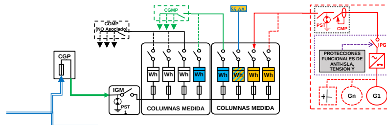
ESQUEMA 95 (Opcional a ESQUEMA 92 con medida en paralelo de Generación Bruta, SS,AA, y Consumo) Colectivo - CON compensación (si Renovable) o Venta Excedentes - en Instalación Enlace Red interior - Finca \geq 2 Suministros - P_{gIE} \leq 50 kW - P_c \leq 50 kW - Modo Dependiente
