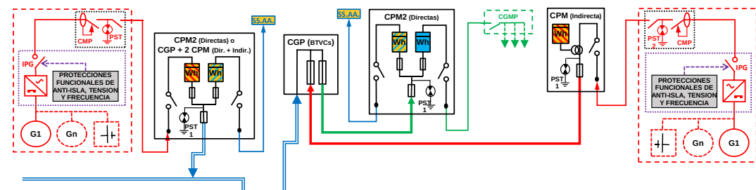
ESQUEMA 73 (Opcional a ESQUEMA 65 con medida en paralelo de Generación Bruta, SS.AA. y Consumo) Individual - CON Venta Excedentes - Mixta: a través Red Distribución y en Instalación Enlace - Finca 1 Suministro - 50 < P_{glE} \leq 100 \text{ kW} - 50 < P_c \leq 400 \text{ kW} - Modo Dependiente
