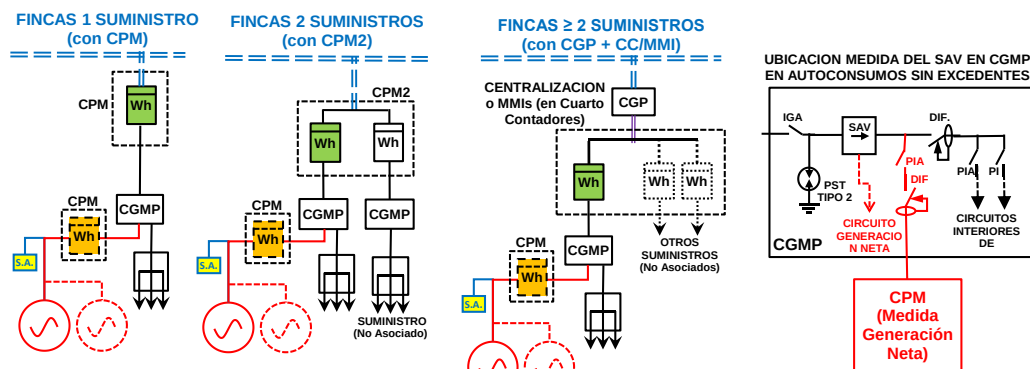
ESQUEMA MEDIDA "B (II)" (Individual en red Interior: en "Serie" en CGMP de instalación interior) (1 Contador bidireccional en Frontera del Consumidor + 1 contador en Generación Neta)
