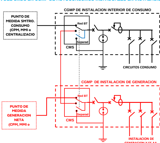
Figura 3. Ubicación del Conmutador a Modo Separado (CMS).
