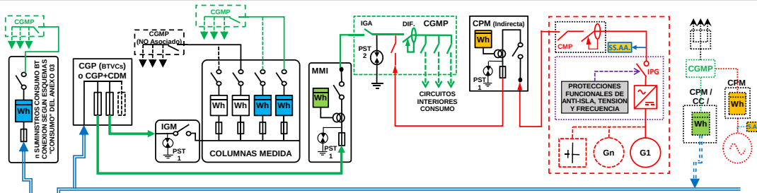
ESQUEMA 104 Colectivo - CON compensación (si Renovable) o Venta Excedentes - Compartida: a través Red Distribución y 100% generación en CGMP instalación interior - Finca \geq 2 Suministros - 50 < P_{gII} \leq 250 \text{ kW} - PCG \leq 250 \text{ kW} - Modo Dependiente
