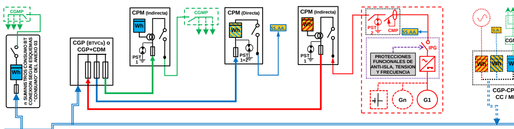
ESQUEMA 115 (Opcional a ESQUEMA 108 con medida en paralelo de Generación Bruta, SS.AA. y Consumo) Colectivo - CON compensación (si Renovable) o Venta Excedentes - Compartida: a través Red Distribución y 100% generación en instalación enlace edificio - Finca 1 Suministro - 50 < P_{gIE} \leq 100 kW - P_c \leq 400 kW - Modo Dependiente
