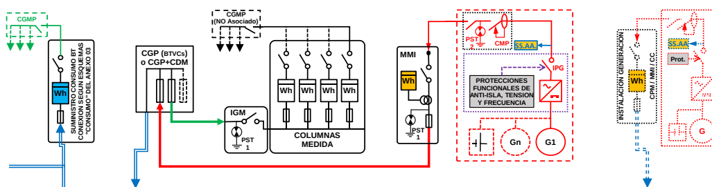
ESQUEMA 48 Individual - CON Venta Excedentes - A través Red Distribución - Finca \geq 2 Suministros - 50 < PgRD \leq 100 kW - P_c \leq 400 kW - Modo Dependiente
