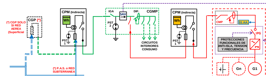
ESQUEMA 8 Individual - SIN Excedentes - en CGMP Red interior - Generación (NO Ren-Co-Res o Distinto Titular o Hibridación) - Finca 1 Suministro - 50 < P_{gII} \leq 400 \text{ kW} - PCG \leq 400 \text{ kW} - Modo
