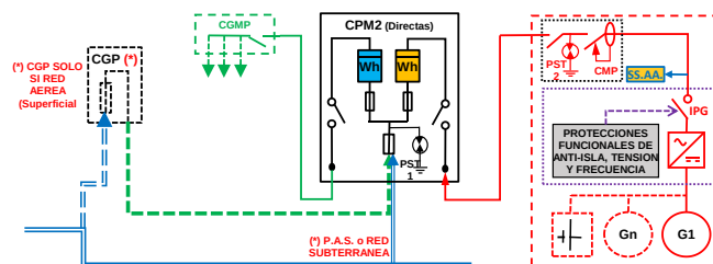
ESQUEMA 27 (Opcional a ESQUEMAS 15 y 20 con medida en paralelo de Generación Neta y Consumo) Individual - CON Venta Excedentes - en Instalación Enlace Red interior - Finca 1 Suministro - P_{gIE} \leq 50 kW - P_c \leq 50 kW - Modo Dependiente
