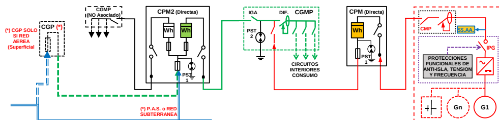
ESQUEMA 23 Individual - CON Venta Excedentes - en CGMP Red interior - Generación (NO Ren-Co-Res o Distinto Titular o Hibridación) - Finca 2 Suministros - P_{gII} \leq 50 \text{ kW} - PCG \leq 50 \text{ kW} - Modo Dependiente
