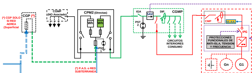
ESQUEMA 3 Individual - SIN Excedentes - en CGMP Red interior - Generación (Ren-Co-Res y mismo Titular) - Finca 2 Suministros - PgII = Cualquiera - PCG ≤ 50 kW - Modo Dependiente
