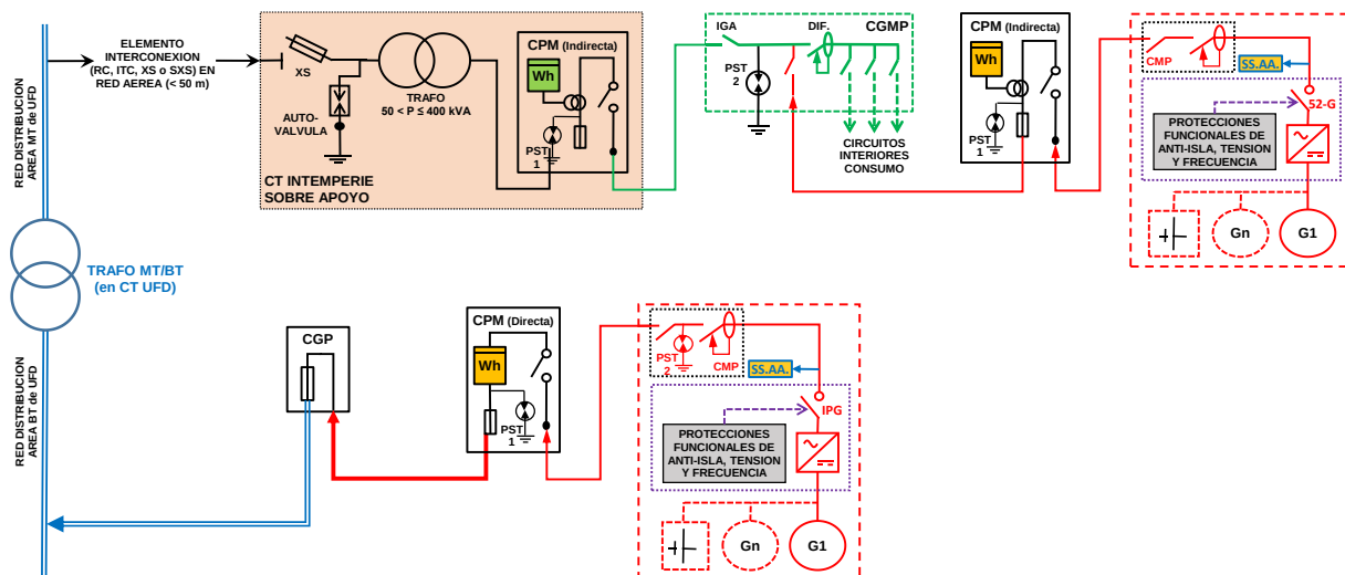
Figura 5. Ejemplo 1 Autoconsumo Combinado (AT/BT).
