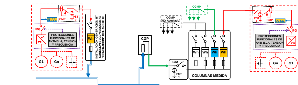
ESQUEMA 67 (Opcional a ESQUEMA 60 con medida en paralelo de Generación Neta y Consumo) Individual - CON Venta Excedentes - Mixta: a través Red Distribución y en Instalación Enlace - Finca \geq 2 Suministros - P_{gIE} \leq 50 kW - 50 < P_c \leq 250 kW - Modo Dependiente
