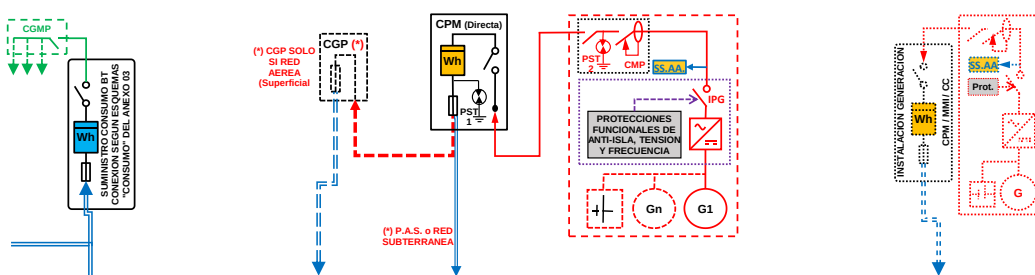
ESQUEMA 43 Individual - CON Venta Excedentes - A través Red Distribución - Conexión directa a red - P_{gRD} \leq 50 \text{ kW} - P_c \leq 400 \text{ kW} - Modo Dependiente
