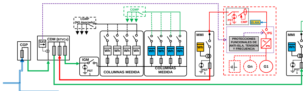
ESQUEMA 85 (Opcional a ESQUEMA 82 con medida en paralelo de Generación Bruta, SS.AA. y Consumo) Colectivo - SIN Excedentes - en Instalación Enlace Red interior - Finca \geq 2 Suministros - P_{gIE} \leq 50 kW - P_c \leq 50 kW - Modo Dependiente
