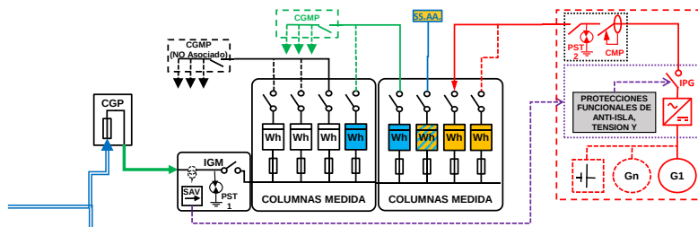
ESQUEMA 85 (Opcional a ESQUEMA 82 con medida en paralelo de Generación Bruta, SS.AA. y Consumo) Colectivo - SIN Excedentes - en Instalación Enlace Red interior - Finca \geq 2 Suministros - P_{gIE} \leq 50 kW - P_c \leq 50 kW - Modo Dependiente
