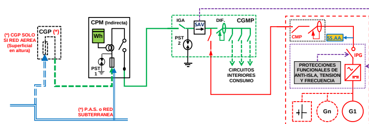
ESQUEMA 2 Individual - SIN Excedentes - en CGMP Red interior - Generación (Ren-Co-Res y mismo Titular) - Finca 1 Suministro - PgII = Cualquiera - 50 < PCG ≤ 400 kW - Modo Dependiente
