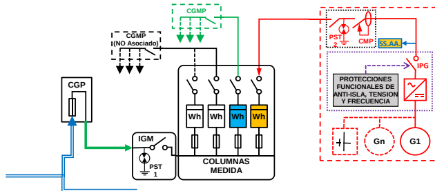
ESQUEMA 31 (Opcional a ESQUEMA 17, 18, 23 y 24 con medida en paralelo de Generación Neta y Consumo) Individual - CON Venta Excedentes - en Instalación Enlace Red interior - Finca \geq 2 Suministros - P_{gIE} \leq 50 kW - P_c \leq 50 kW - Modo Dependiente
