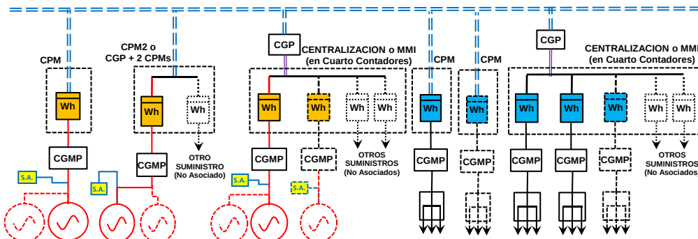
ESQUEMA MEDIDA "C (CR)" (Colectivo a través de Red de distribución) (1 Contador bidireccional en Frontera de cada consumidor + 1 contador en cada Generación Neta en CPM)
