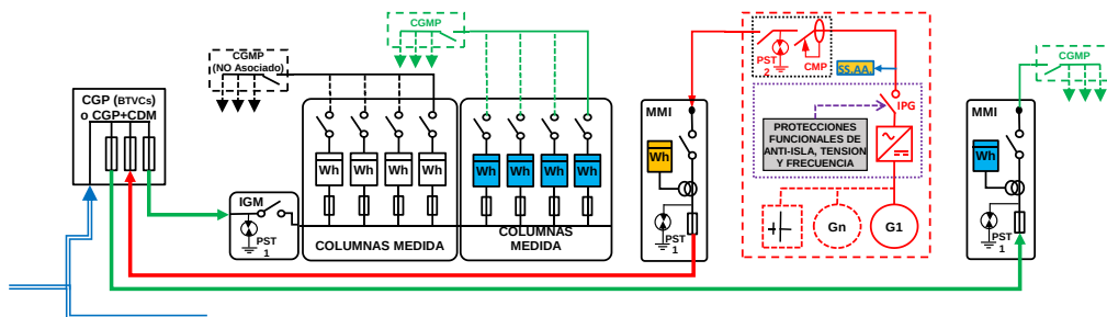
ESQUEMA 94 (Opcional a ESQUEMA 91 con medida en paralelo de Generación Neta y Consumo) Colectivo - CON compensación (si Renovable) o Venta Excedentes - en Instalación Enlace Red interior - Finca \geq 2 Suministros - 50 < P_{gIE} \leq 100 kW - P_c \leq 250 kW - Modo Dependiente
