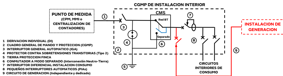
FIGURA MS3 - CONMUTACION MODO SEPARADO EN AUTOCONSUMOS INDIVIDUALES CON GENERACION CONECTADA EN INSTALACION DE ENLACE
