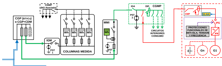
ESQUEMA 19 Individual - CON Compensación Excedentes - en CGMP Red interior - Generación (Renovable y mismo titular) - Finca \geq 2 Suministros - 50 < P_{gII} \leq 100 \text{ kW} ó 50 < P_{CG} \leq 250 \text{ kW} - Modo Dependiente
