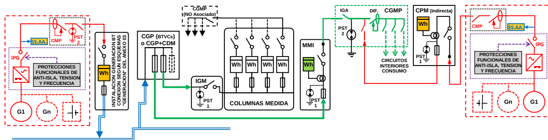
ESQUEMA 61 Individual - CON Venta Excedentes - Mixta: a través Red Distribución y en CGMP Red interior - Finca \geq 2 Suministros - 50 < P_{gIE} \leq 100 kW - PCG \leq 250 kW - Modo Dependiente
