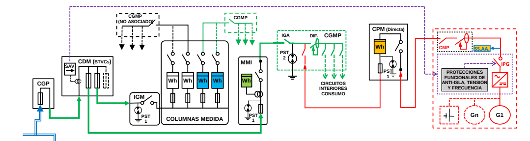
ESQUEMA 80 Colectivo - SIN Excedentes - en CGMP Red interior - Finca \geq 2 Suministros - P_{gII} \leq 50 kW - 50 < PCG \leq 250 kW - Modo Dependiente
