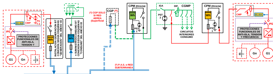
ESQUEMA 132 Colectivo - CON Venta Excedentes - Mixta: a través Red Distribución y en CGMP Red interior - Finca 1 Suministro - P_{glt} \leq 50 kW - 50 < PCG \leq 400 kW - Modo Dependiente
