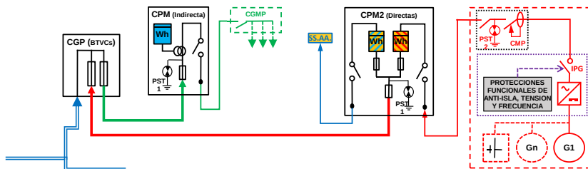
ESQUEMA 36 (Opcional a ESQUEMA 28 con medida en paralelo de Generación Bruta, SS.AA. y Consumo) Individual - CON Venta Excedentes - en Instalación Enlace Red interior - Finca 1 Suministro - PgIe ≤ 50 kW - 50 < Pc ≤ 400 kW - Modo Dependiente
