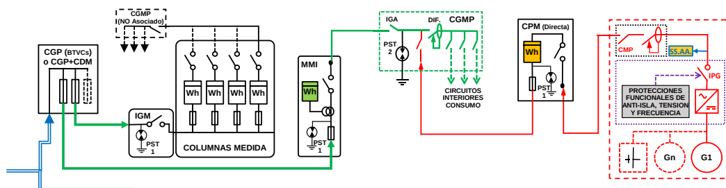
ESQUEMA 25 Individual - CON Venta Excedentes - en CGMP Red interior - Generación (NO Ren-Co-Res o Distinto Titular o Hibridación) - Finca \geq 2 Suministros - P_{gII} \leq 50 \text{ kW} - 50 < PCG \leq 250 \text{ kW} - Modo Dependiente
