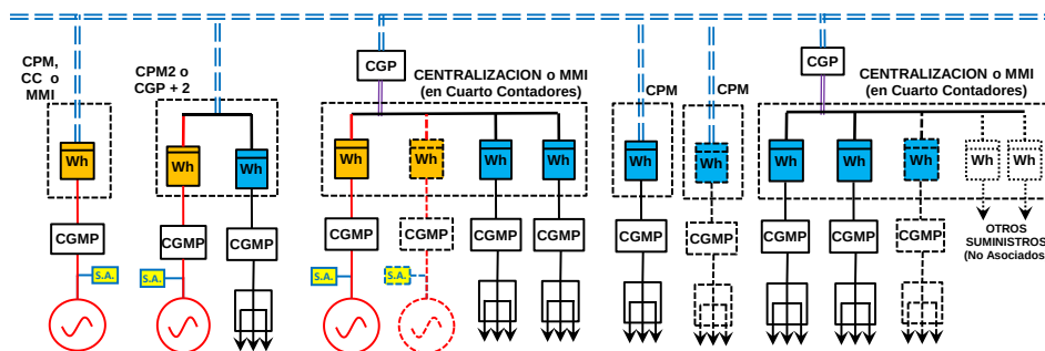
ESQUEMA MEDIDA "C (CM)" (Colectivo Mixto: a través red distribución y en "Paralelo" en instalación de enlace) (1 Contador bidireccional en Frontera de cada consumidor + 1 contador en cada Generación Neta en CPM)
