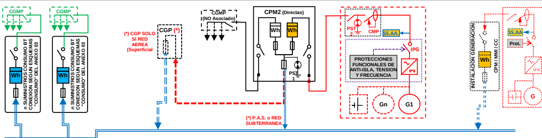
ESQUEMA 121 Colectivo - CON Venta Excedentes - A través Red Distribución - Finca 1 Suministro - P_{gIE} \leq 50 \text{ kW} - P_c \leq 400 \text{ kW} - Modo Dependiente
