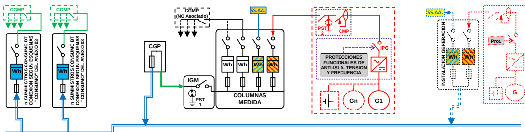
ESQUEMA 129 (Opcional a ESQUEMA 123 con medida en paralelo de Generación Bruta, SS.AA. y Consumo) Colectivo - CON Venta Excedentes - A través Red Distribución - Finca \geq 2 Suministros - P_{gIE} \leq 50 \text{ kW} - P_c \leq 400 \text{ kW} - Modo Dependiente
