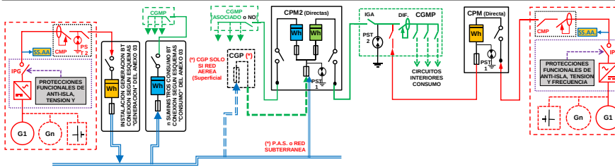
ESQUEMA 135 Colectivo - CON Venta Excedentes - Mixta: a través Red Distribución y en CGMP Red interior - Finca \geq 2 Suministros - P_{glt} \leq 50 kW - PCG \leq 50 kW - Modo Dependiente
