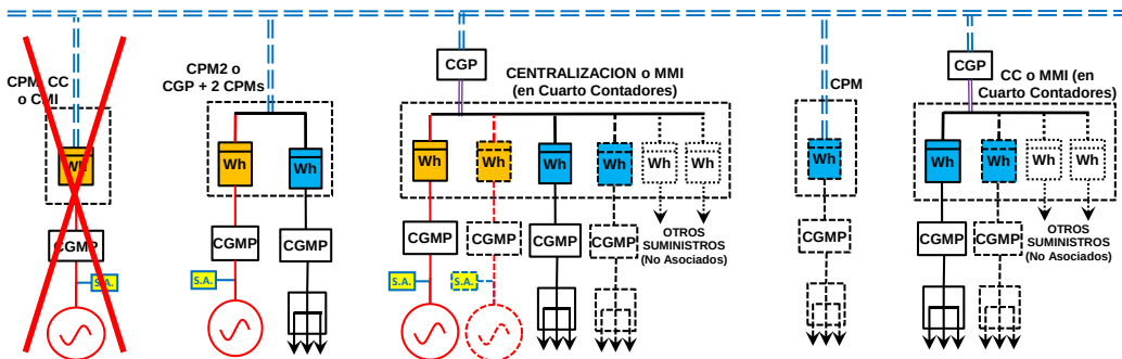
ESQUEMA MEDIDA "C (CC)" (Colectivo Compartido: a través red y en "Paralelo" en instalación enlace) (1 Contador bidireccional en Frontera de cada consumidor + 1 contador en cada Generación Neta en instalación enlace)
