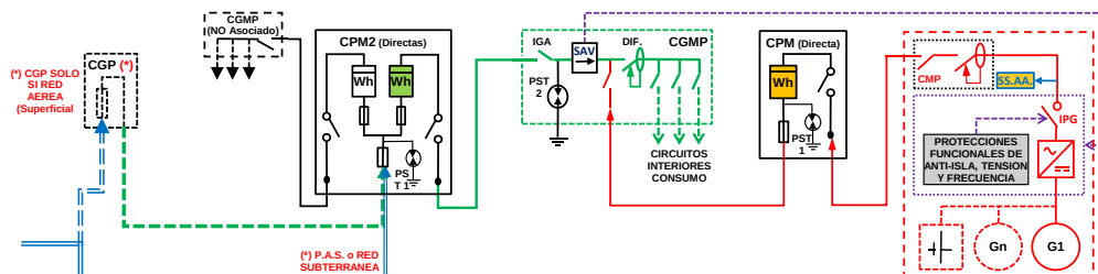
ESQUEMA 10 Individual - SIN Excedentes - en CGMP Red interior - Generación (NO Ren-Co-Res o Distinto Titular o Hibridación) - Finca 2 Suministros - P_{gII} \leq 50 \text{ kW} - PCG \leq 50 \text{ kW} - Modo
