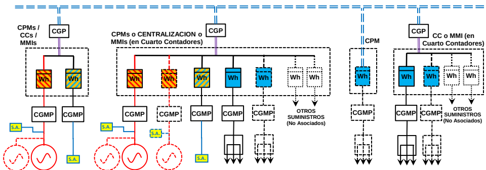
ESQUEMA MEDIDA "D (CM)" (Colectivo Mixto: a través red distribución y en "Paralelo" en instalación de enlace) (1 Contador bidireccional en Frontera de cada consumidor + 1 contador en cada Generación Bruta + 1 contador en cada SS.AA.)
