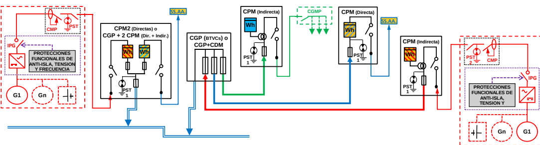
ESQUEMA 73 (Opcional a ESQUEMA 65 con medida en paralelo de Generación Bruta, SS.AA. y Consumo) Individual - CON Venta Excedentes - Mixta: a través Red Distribución y en Instalación Enlace - Finca 1 Suministro - 50 < P_{glE} \leq 100 \text{ kW} - 50 < P_c \leq 400 \text{ kW} - Modo Dependiente
