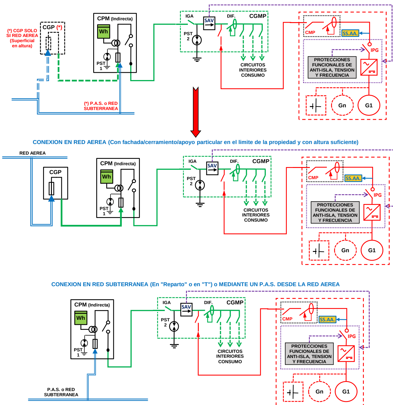
Figura 9. Esquemas de conexión en red aérea o subterránea.
