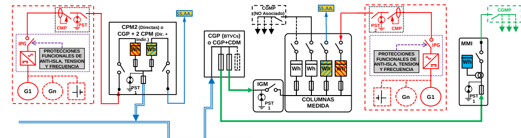
ESQUEMA 75 (Opcional a ESQUEMA 67 con medida en paralelo de Generación Bruta, SS.AA. y Consumo) Individual - CON Venta Excedentes - Mixta: a través Red Distribución y en Instalación Enlace - Finca \geq 2 Suministros - P_{glE} \leq 50 \text{ kW} - 50 < P_c \leq 250 \text{ kW} - Modo Dependiente
