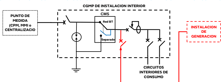
UBICACION DEL CMDS EN CGMP DE AUTOCONSUMOS INDIVIDUALES EN INSTALACION INTERIOR CON EXCEDENTES
