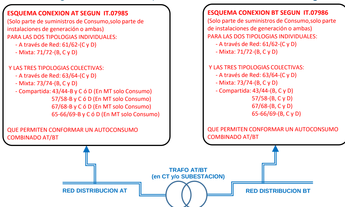
Figura 4. Conexión de Autoconsumos Combinados (AT/BT).
