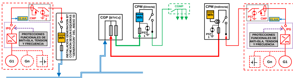
ESQUEMA 64 (Opcional a ESQUEMA 57 (Si PCG \leq 50 kW) con medida en paralelo de Generación Neta y Consumo) Individual - CON Venta Excedentes - Mixta: a través Red Distribución y en Instalación Enlace - Finca 1 Suministro - 50 < P_{gIE} \leq 100 kW - P_c \leq 50 kW - Modo Dependiente
