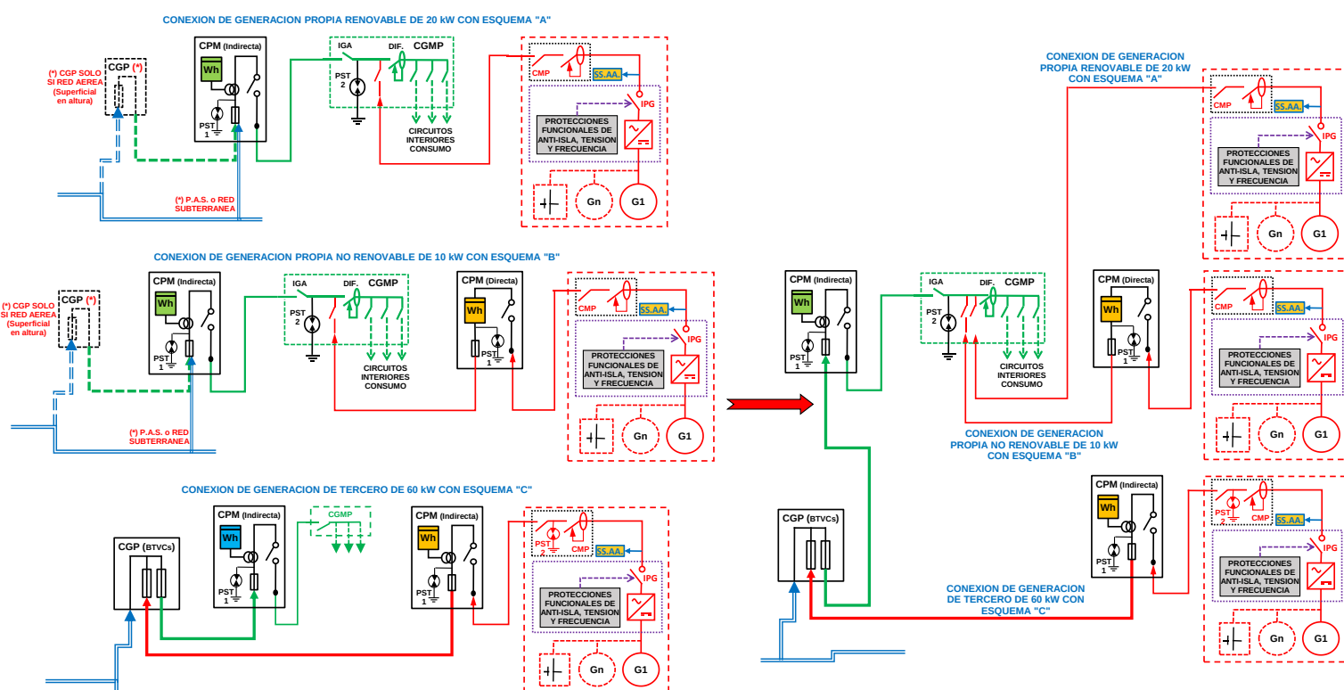
Figura 10. Ejemplo 1 Autoconsumo con varias instalaciones de generación según algunos de los distintos esquemas de medida aceptados para su “Tipología”.
