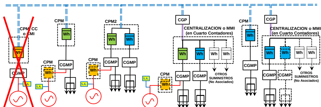
ESQUEMA MEDIDA "B (CC)" (Colectivo Compartido: a través red y en "Serie" en CGMP suministro con generación) (1 Contador bidireccional en Frontera de cada consumidor + 1 contador en cada Generación Neta en CPM)
