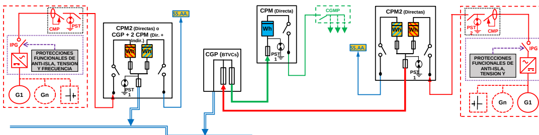
ESQUEMA 70 (Opcional a ESQUEMA 62 con medida en paralelo de Generación Bruta, SS.AA. y Consumo) Individual - CON Venta Excedentes - Mixta: a través Red Distribución y en Instalación Enlace - Finca 1 Suministro - P_{gIE} \leq 50 kW - P_c \leq 50 kW - Modo Dependiente
