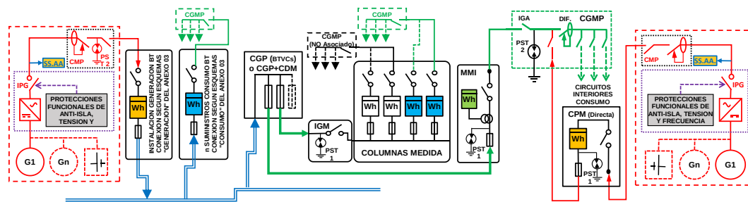
ESQUEMA 137 Colectivo - CON Venta Excedentes - Mixta: a través Red Distribución y en CGMP Red interior - Finca \geq 2 Suministros - 50 < P_{gII} \leq 100 \text{ kW} - PCG \leq 250 \text{ kW} - Modo Dependiente
