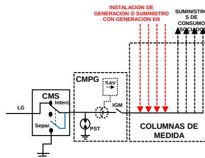
UBICACION DEL CMDS ANTES DE CENTRALIZACION EN AUTOCONSUMOS COLECTIVOS
