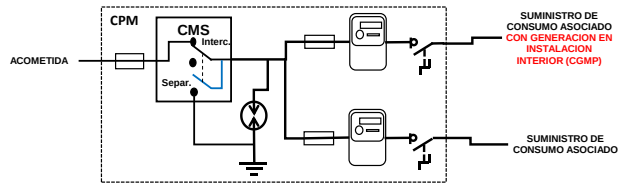
FIGURA M56 - CONMUTACION MODO SEPARADO EN AUTOCONSUMOS COLECTIVOS CON GENERACION EN CC
