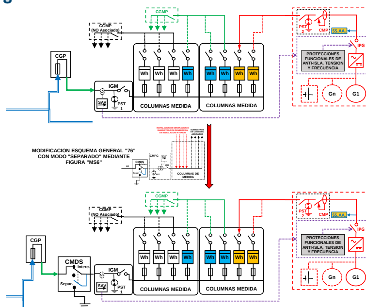
Figura 7. Modificación del esquema de conexión para funcionamiento “Separado”.
