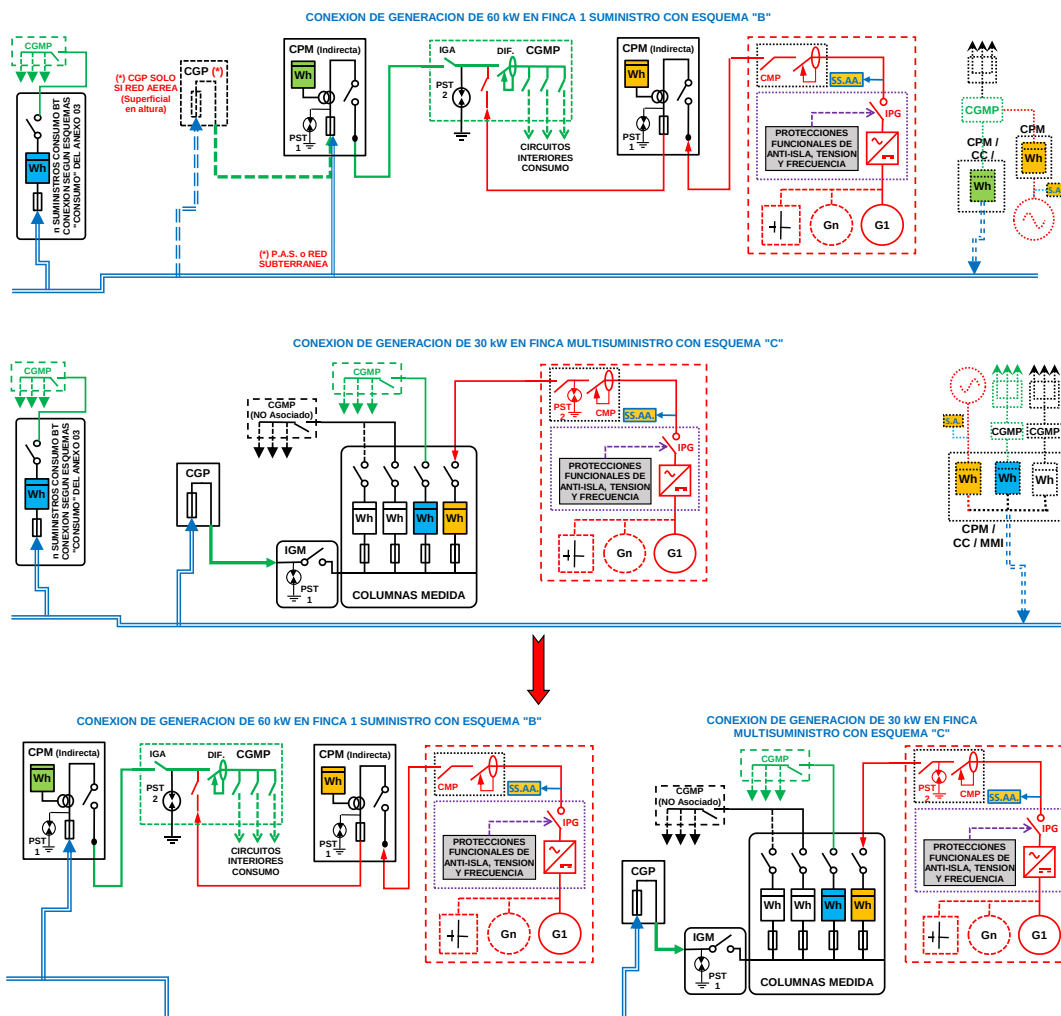
Figura 11. Ejemplo 2 Autoconsumo con varias instalaciones de generación según algunos de los distintos esquemas de medida aceptados para su “Tipología”.
