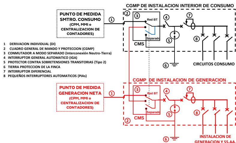
FIGURA MS3 - CONMUTACION MODO SEPARADO EN AUTOCONSUMOS INDIVIDUALES CON GENERACION CONECTADA EN INSTALACION DE ENLACE
