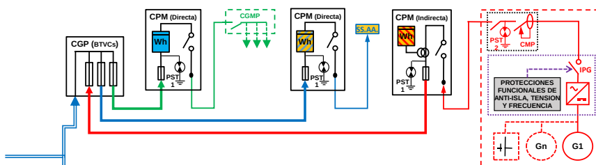
ESQUEMA 37 (Opcional a ESQUEMA 29 con medida en paralelo de Generación Bruta, SS.AA. y Consumo) Individual - CON Venta Excedentes - en Instalación Enlace Red interior - Finca 1 Suministro - 50 < PglE ≤ 100 kW - Pc ≤ 50 kW - Modo Dependiente
