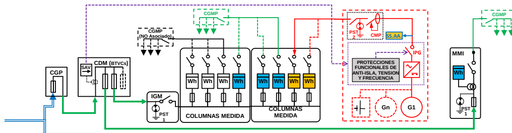
ESQUEMA 84 (Opcional a ESQUEMA 81 con medida en paralelo de Generación Neta y Consumo) Colectivo - SIN Excedentes - en Instalación Enlace Red interior - Finca \geq 2 Suministros - 50 < P_{gIE} \leq 250 kW - P_c \leq 250 kW - Modo Dependiente
