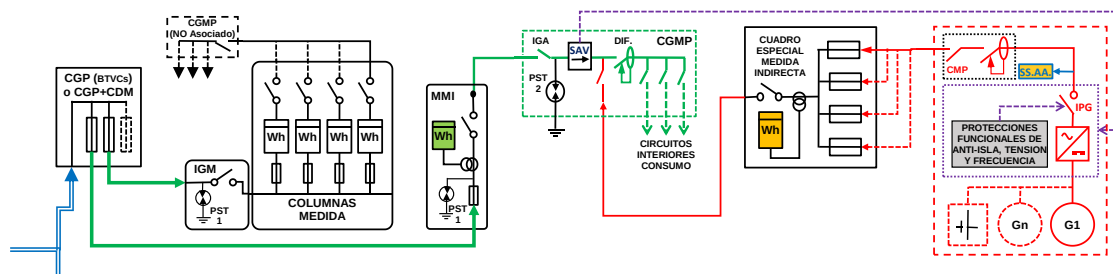
ESQUEMA 14 Individual - SIN Excedentes - en CGMP Red interior - Generación (NO Ren-Co-Res o Distinto Titular o Hibridación) - Finca \geq 2 Suministros - P_{gII} > 250 kW - PCG \leq 250 kW - Modo
