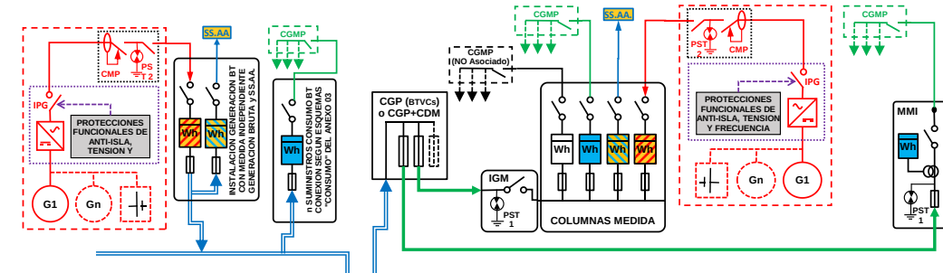
ESQUEMA 150 (Opcional a ESQUEMAS 143 con medida en paralelo de Generación Bruta, SS.AA. y Consumo) Colectivo - CON Venta Excedentes - Mixta: a través Red Distribución y en Instalación Enlace - Finca ≥ 2 Suministros - PglE ≤ 50 kW - Pc ≤ 250 kW - Modo Dependiente
