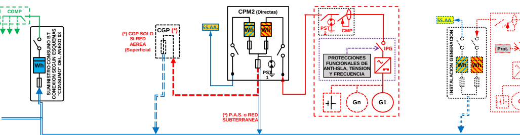
ESQUEMA 50 (Opcional a ESQUEMA 44 con medida en paralelo de Generación Bruta, SS.AA. y Consumo) Individual - CON Venta Excedentes - A través Red Distribución - Conexión directa a red - 50 < PgRD \leq 100 kW - P_c \leq 400 kW - Modo Dependiente
