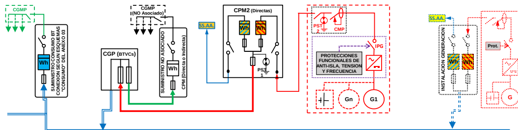
ESQUEMA 51 (Opcional a ESQUEMA 45 con medida en paralelo de Generación Bruta, SS.AA. y Consumo) Individual - CON Venta Excedentes - A través Red Distribución - Finca 1 Suministro - PgRD ≤ 50 kW - Pc ≤ 400 kW - Modo Dependiente
