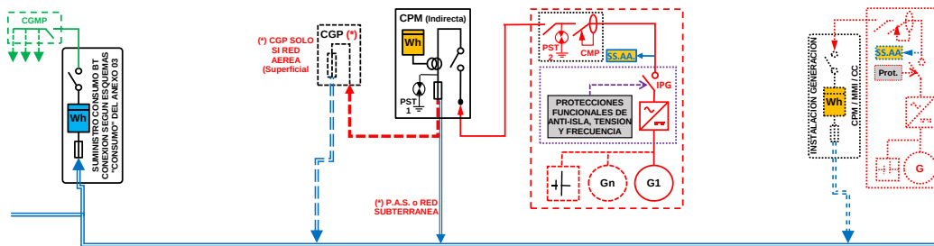
ESQUEMA 45 Individual - CON Venta Excedentes - A través Red Distribución - Finca 1 Suministro - P_{gRD} \leq 50 \text{ kW} - P_c \leq 400 \text{ kW} - Modo Dependiente
