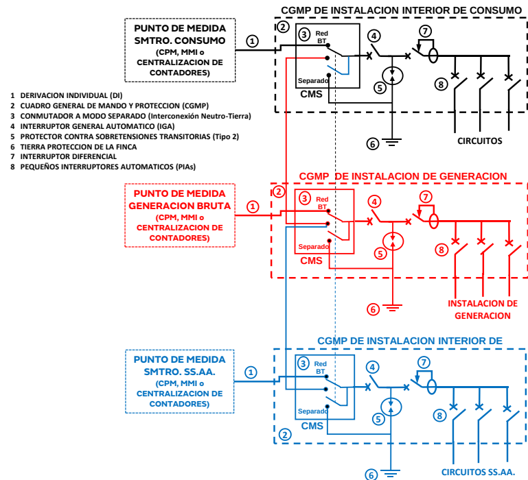
FIGURA M55 - CONMUTACION MODO SEPARADO EN AUTOCONSUMOS COLECTIVOS CON GENERACION EN CPMs
