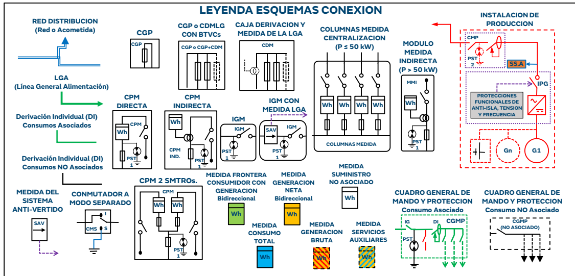
FIGURA MS1 - CONMUTACION MODO SEPARADO EN AUTOCONSUMO INDIVIDUAL SIN EXCEDENTES CON GENERACION CONECTADA EN CGMP INSTALACION INTERIOR
