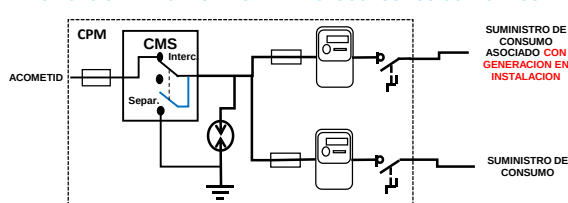
UBICACION DEL CMDS EN CPM DE AUTOCONSUMOS COLECTIVOS
