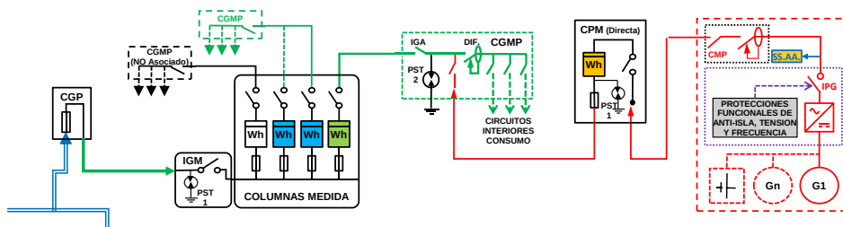
ESQUEMA 89 Colectivo - CON compensación (si Renovable) o Venta Excedentes - en CGMP Red interior - Finca \geq 2 Suministros - P_{gII} \leq 50 kW - PCG \leq 50 kW - Modo Dependiente
