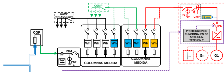
ESQUEMA 82 (Opcional a ESQUEMA 78 ó 79 con medida en paralelo de Generación Neta y Consumo) Colectivo - SIN Excedentes - en Instalación Enlace Red interior - Finca \geq 2 Suministros - P_{gIE} \leq 50 kW - P_c \leq 50 kW - Modo Dependiente
