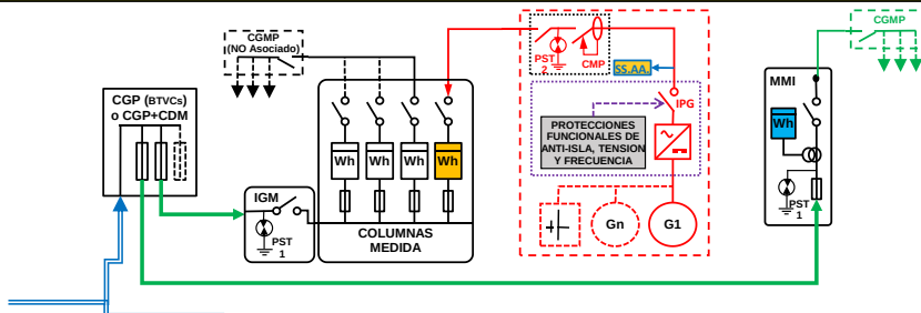
ESQUEMA 32 (Opcional a ESQUEMAS 19 (Si P_{gII} \leq 50 kW) y 25 con medida en paralelo de Generación Neta y Consumo) Individual - CON Venta Excedentes - en Instalación Enlace Red interior - Finca \geq 2 Suministros - P_{gIE} \leq 50 kW - 50 < P_c \leq 250 kW - Modo Dependiente
