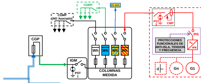
ESQUEMA 39 (Opcional a ESQUEMA 31 con medida en paralelo de Generación Bruta, SS.AA. y Consumo) Individual - CON Venta Excedentes - en Instalación Enlace Red interior - Cualquier Finca - PglE ≤ 50 kW - Pc ≤ 50 kW - Modo Dependiente
