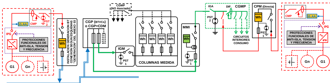
ESQUEMA 60 Individual - CON Venta Excedentes - Mixta: a través Red Distribución y en CGMP Red interior - Finca ≥ 2 Suministros - PglI ≤ 50 kW - 50 < PCG ≤ 250 kW - Modo Dependiente
