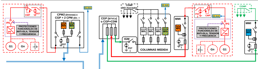
ESQUEMA 78 Colectivo - SIN Excedentes - en CGMP Red interior - Finca 2 Suministros - P_{gII} \leq 50 kW - PCG \leq 50 kW - Modo Dependiente
