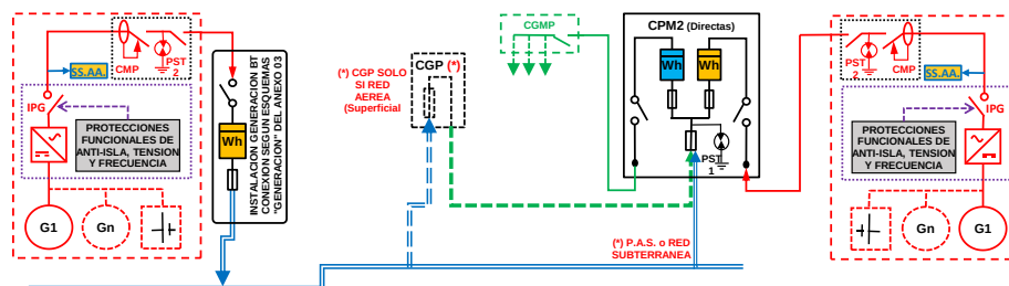
ESQUEMA 62 (Opcional a ESQUEMA 55 con medida en paralelo de Generación Neta y Consumo) Individual - CON Venta Excedentes - Mixta: a través Red Distribución y en Instalación Enlace - Finca 1 Suministro - P_{gIE} \leq 50 kW - P_c \leq 50 kW - Modo Dependiente
