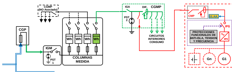
ESQUEMA 18 Individual - CON Compensación Excedentes - en CGMP Red interior - Generación (Renovable y mismo titular) - Finca \geq 2 Suministros - P_{gII} \leq 50 \text{ kW} - P_{CG} \leq 50 \text{ kW} - Modo Dependiente
