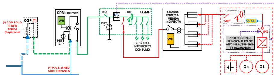
ESQUEMA 9 Individual - SIN Excedentes - en CGMP Red interior - Generación (NO Ren-Co-Res o Distinto Titular o Hibridación) - Finca 1 Suministro - P_{gII} > 400 \text{ kW} - PCG \leq 400 \text{ kW} - Modo
