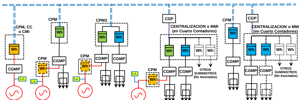
ESQUEMA MEDIDA "B (CM)" (Colectivo Mixto: a través red distribución y en "Serie" en CGMP) (1 Contador bidireccional en Frontera de cada consumidor + 1 contador en cada Generación Neta en CPM)
