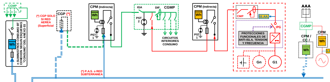
ESQUEMA 100 Colectivo - CON compensación (si Renovable) o Venta Excedentes - Compartida: a través Red Distribución y 100% generación en CGMP instalación interior - Finca 1 Suministro - 50 < P_{gII} \leq 100 kW - PCG \leq 400 kW - Modo Dependiente
