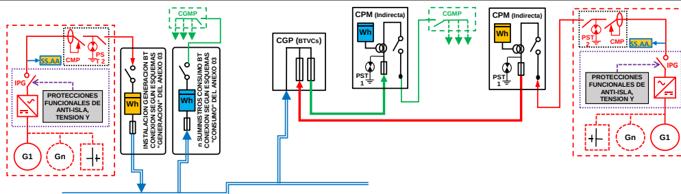
ESQUEMA 142 (Opcional a ESQUEMAS 134 ó 135 con medida en paralelo de Generación Neta y Consumo) Colectivo - CON Venta Excedentes - Mixta: a través Red Distribución y en Instalación Enlace - Finca \geq 2 Suministros - P_{glE} \leq 50 kW - P_c \leq 50 kW - Modo Dependiente
