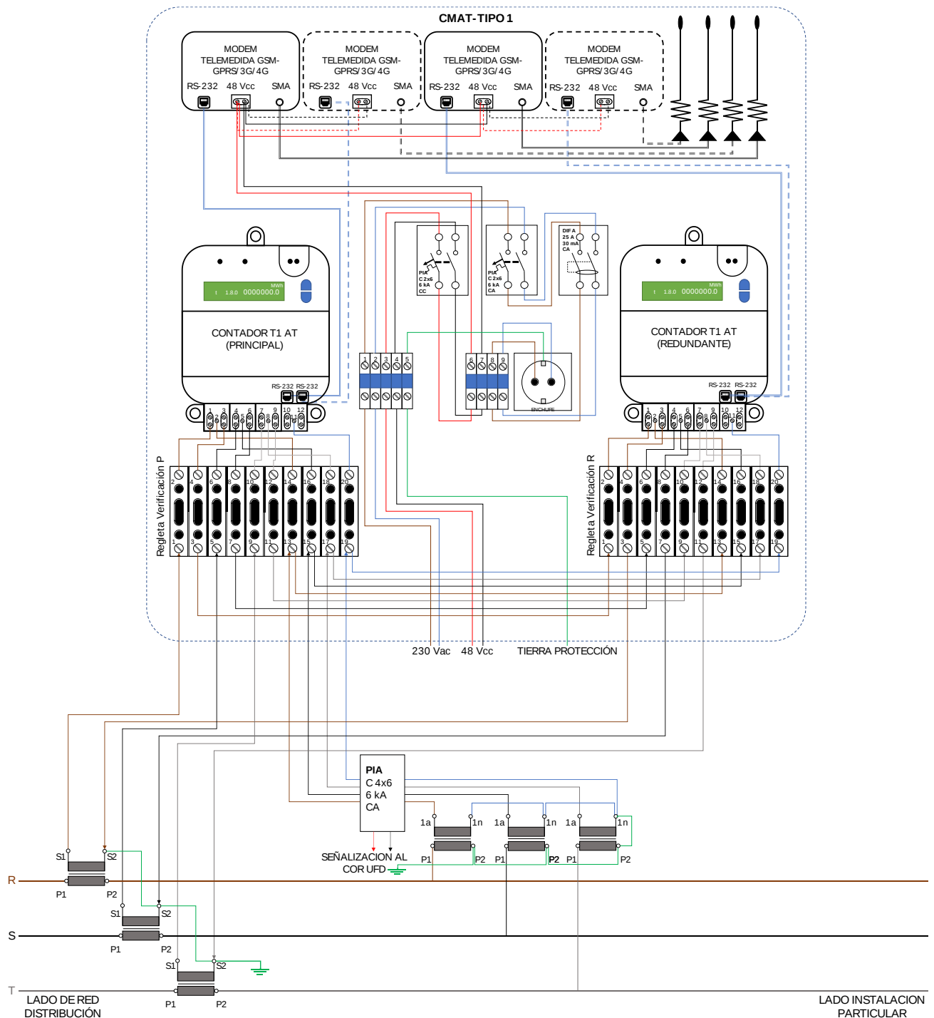
Figura 9. AT-P+R(c) Medida Principal+Redundante > 36 kV sin cajas de centralización
