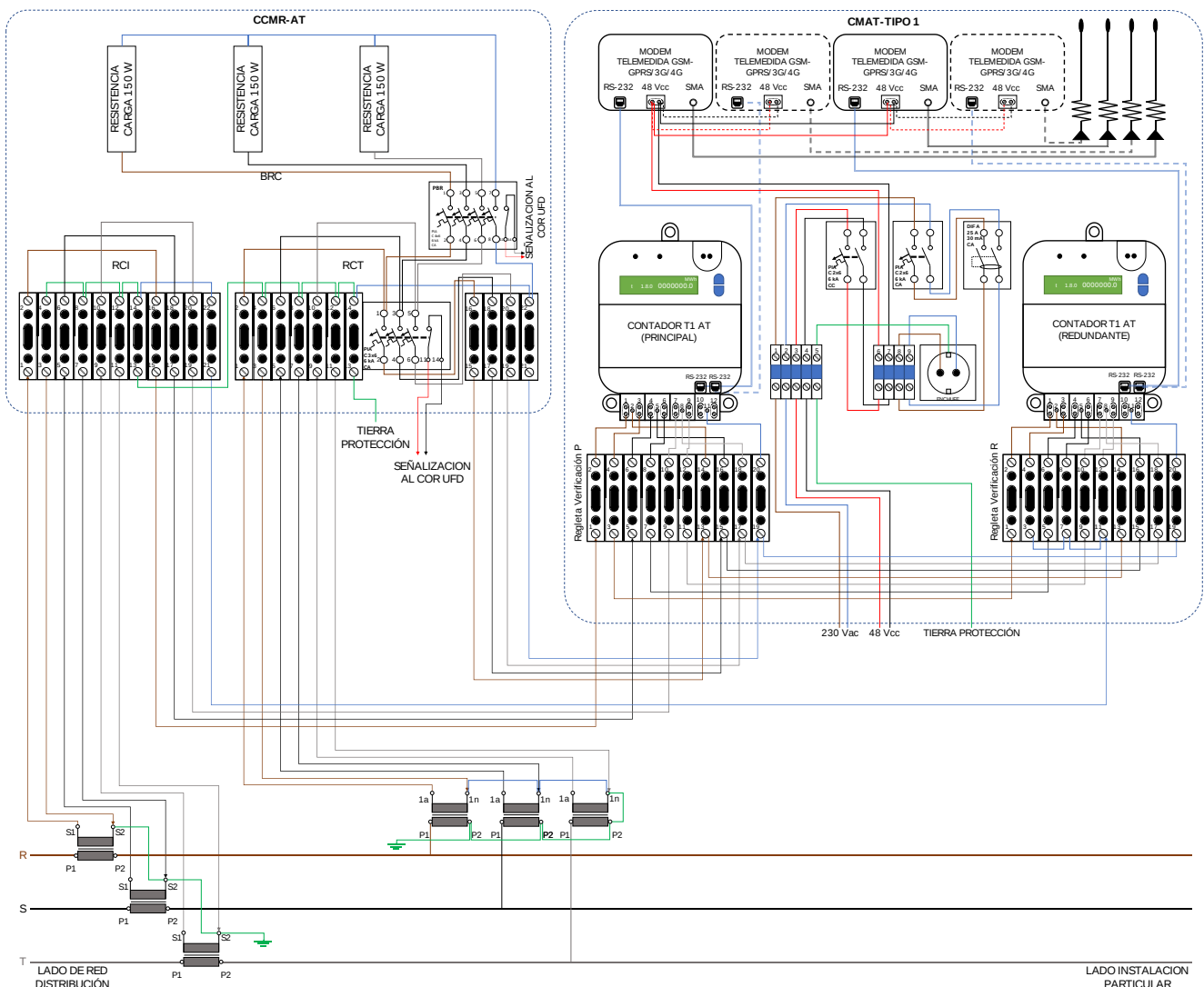
Figura 11. AT-P+R(e) Medida Principal+Redundante > 36 \text{ kV} con centralización de tensiones e intensidades en CCMR
