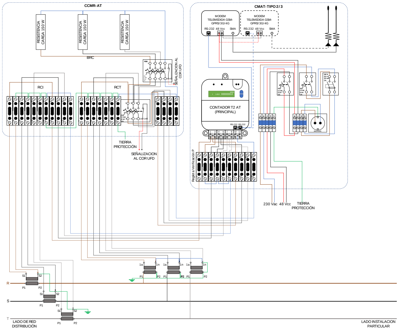
Figura 7. AT-P(e) Medida Principal > 36 kV con centralización de tensiones e intensidades en CCMR
