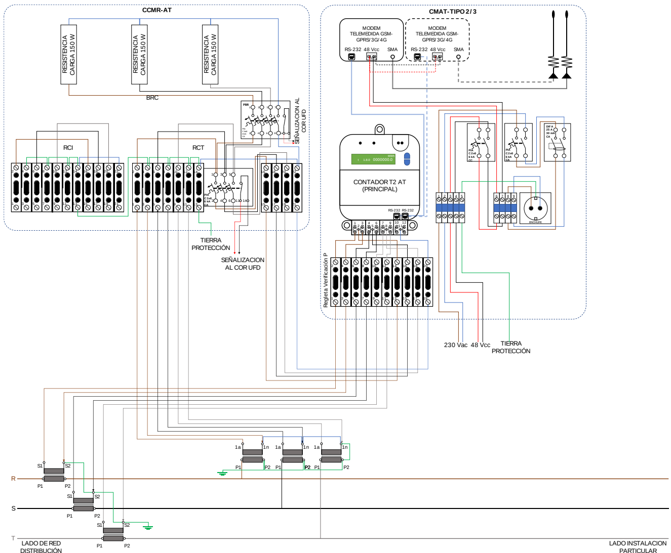
Figura 6. AT-P(d) Medida Principal > 36 kV con Resistencias en CCMR
