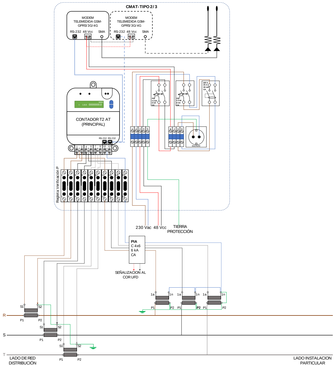
Figura 5. AT-P(c) Medida Principal > 36 kV sin cajas de centralización
