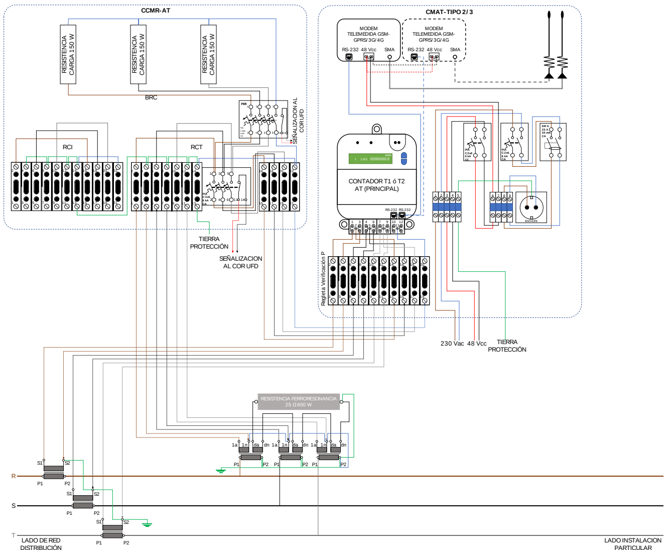
Figura 2. AT-P(b) Medida Principal \leq 36 \text{ kV} con Resistencias en CCMR
