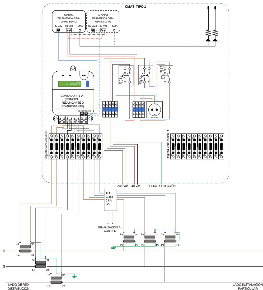
Figura 13. AT-P+[R/C](a) Medida Principal o Redundante/Comprobante > 36 kV sin cajas de centralización
