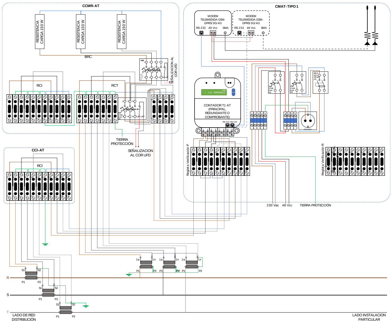
Figura 16. AT-P+[R/C](d) Medida Principal o Redundante/ Comprobante > 36 \text{ kV} con CCMR y CCI
