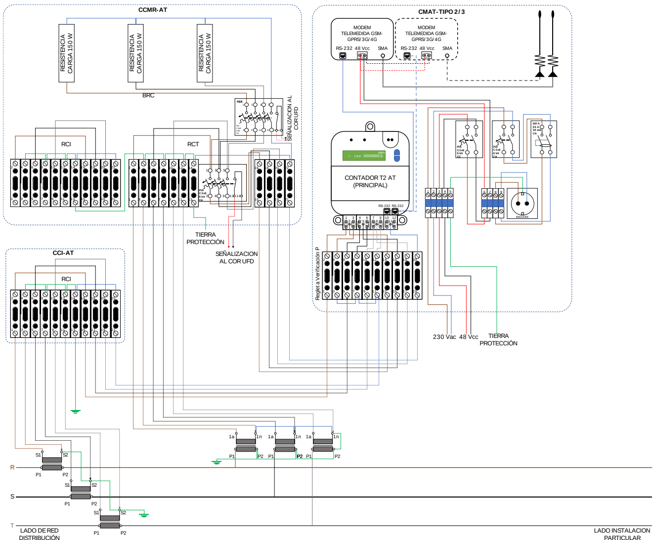
Figura 8. AT-P(f) Medida Principal > 36 \text{ kV} con CCMR y CCI
