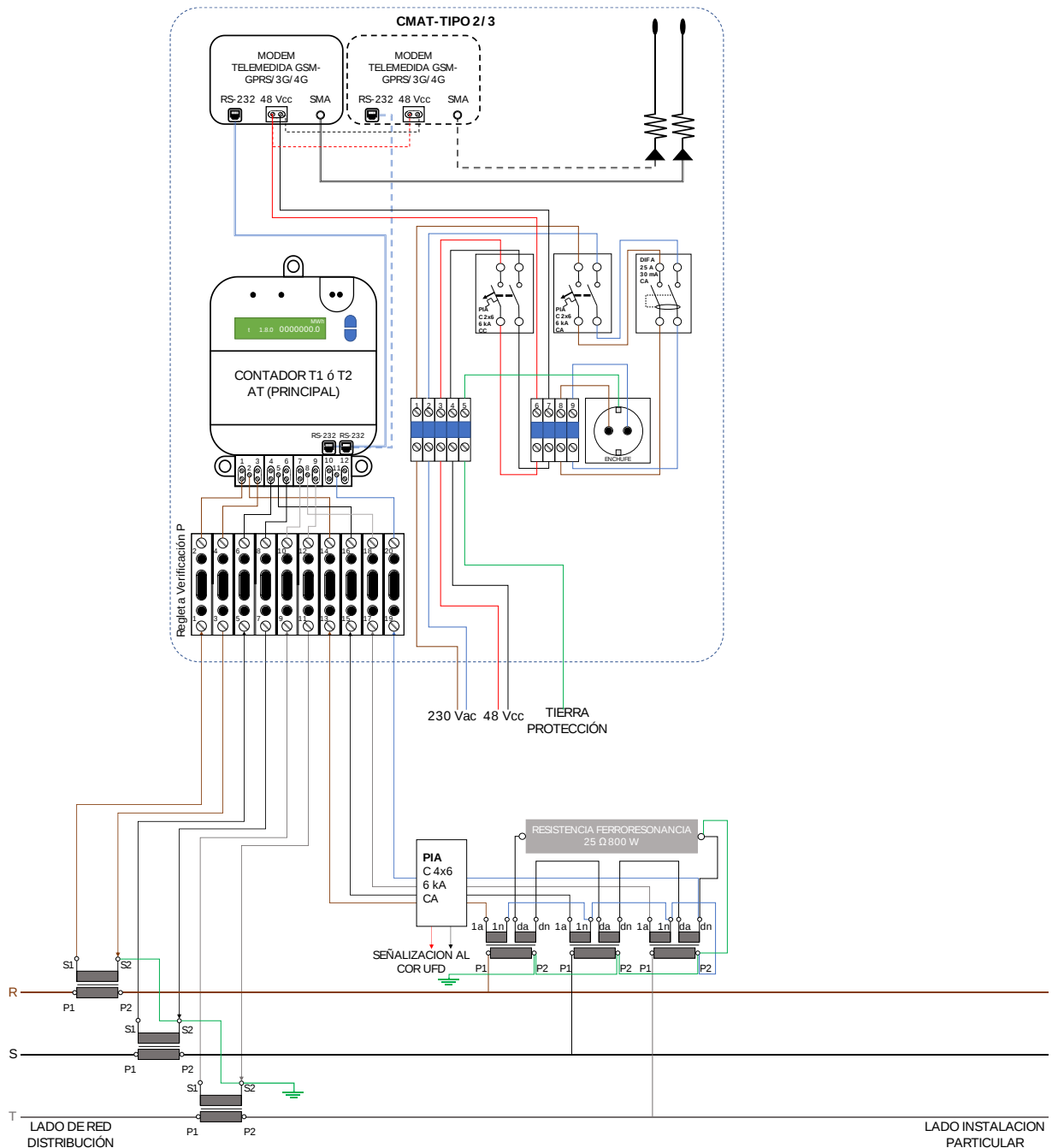
Figura 1. AT-P(a) Medida Principal \leq 36 kV sin cajas de centralización
