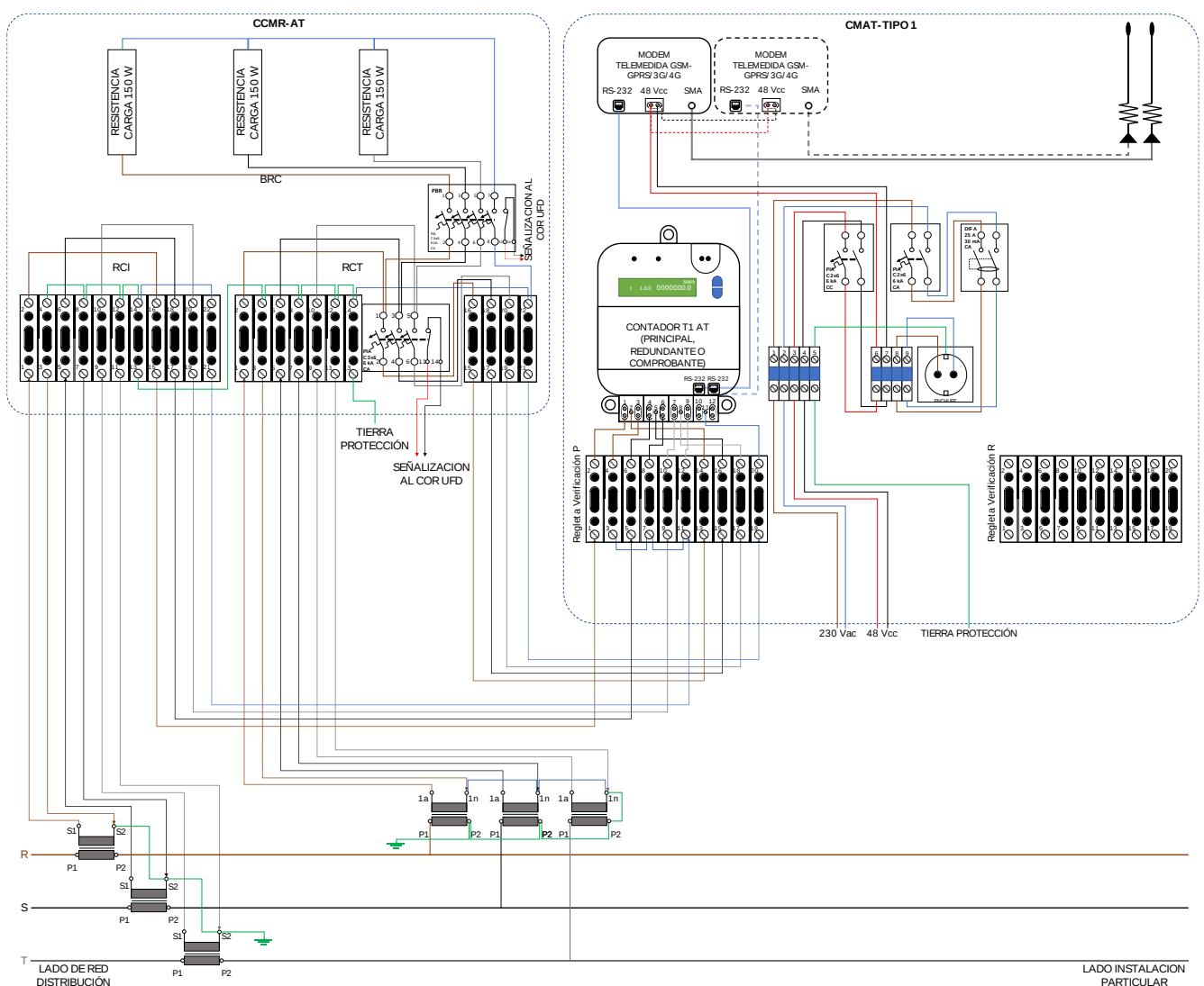
Figura 15. AT-P+[R/C](c) Medida Principal o Redundante/Comprobante > 36 \text{ kV} con centralización de tensiones e intensidades en CCMR
