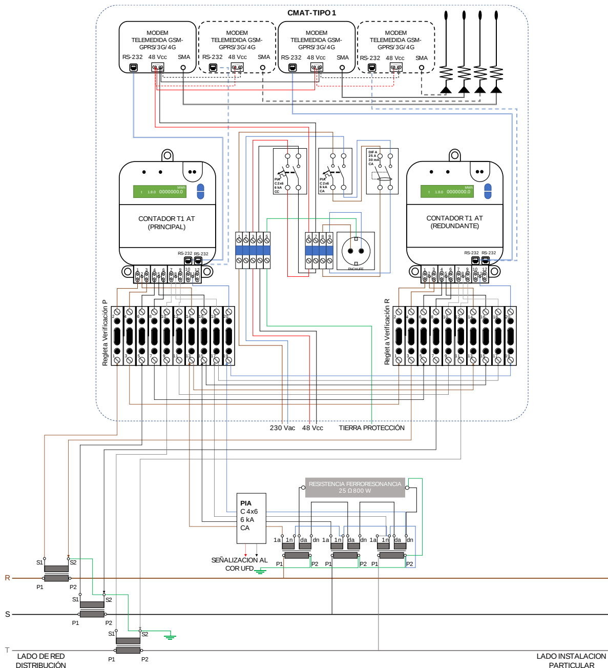
Figura 3. AT-P+R(a) Medida Principal+Redundante \leq 36 kV sin cajas de centralización
